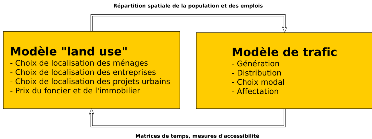
FIGURE 7.8 – Schéma simplifié d'un modèle dynamique de type LUTI. D'après le rapport final sur la première phase d'ULTISIM [61].
