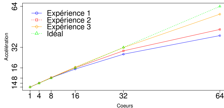
FIGURE 4.10 – Accélération de la simulation SkelGIS pour les trois expériences.
