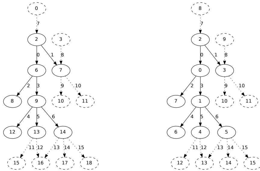
(a) Partie du graphe global qui intéresse le processeur 1 pour gérer ses données locales et les voisinages nécessaires.
