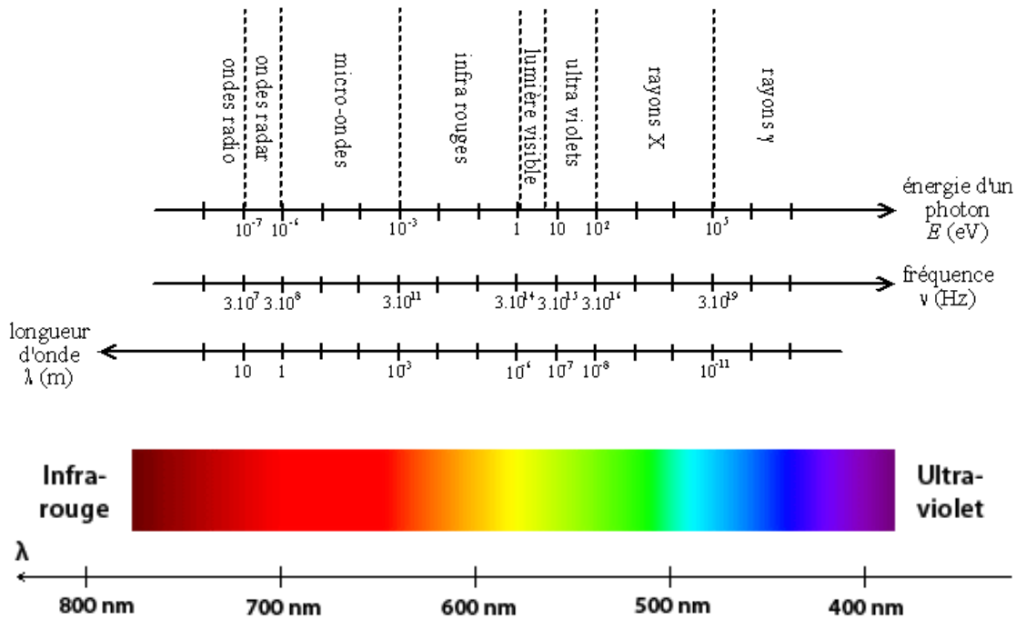
Figure 1.2.1 – Spectre électromagnétique. Haut : classement des ondes électromagnétiques par longueur d'onde, fréquence et énergie des photons (wikipedia.org). Bas : spectre électromagnétique visible. Les couleurs correspondent à la couleur perçue par un observateur humain "standard" pour une lumière monochromatique de longueur d'onde donnée.
