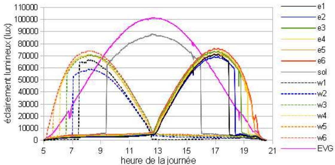
Figure IV-1 : Éclairements lumineux mesurés sur la maquette pour H/W=0,5 avec les façades noires le 22/06/12
