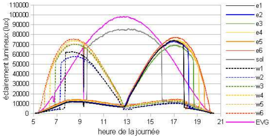
Figure IV-3 : Éclairages lumineux mesurés sur la maquette pour H/W=0,5 avec les façades en crépi le 17/07/12
