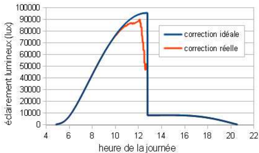
Figure III-56 : Éclairement lumineux modélisé pour un plan vertical orienté vers l'est, avec une correction en cosinus idéale et réelle
