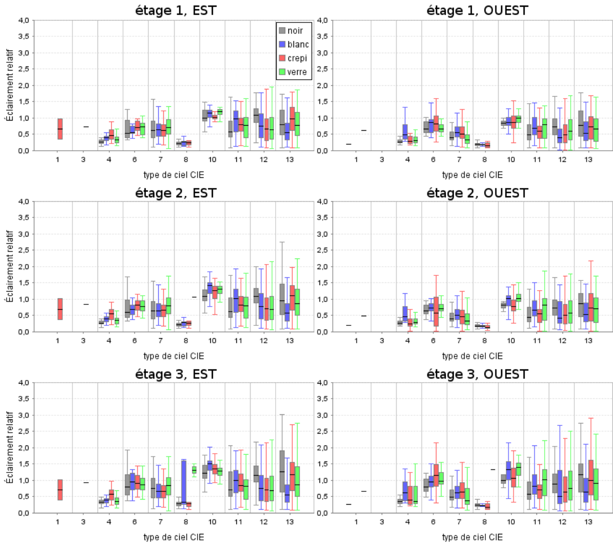
Figure IV-42 : Éclaircement relatif pour les étages 1 à 3 des façades Est et Ouest, avec H/W=0,5 pour les situations avec soleil visible
