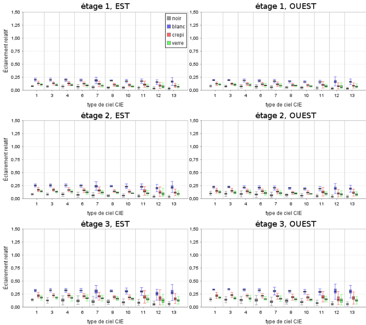
Figure IV-35 : Éclaircement relatif pour les étages 1 à 3 des façades Est et Ouest, avec H/W=2 pour les situations sans soleil visible
