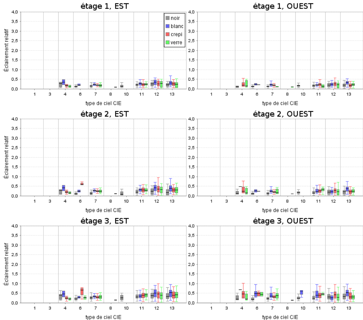
Figure IV-46 : Éclairage relatif pour les étages 1 à 3 des façades Est et Ouest, avec H/W=2 pour les situations avec soleil visible
