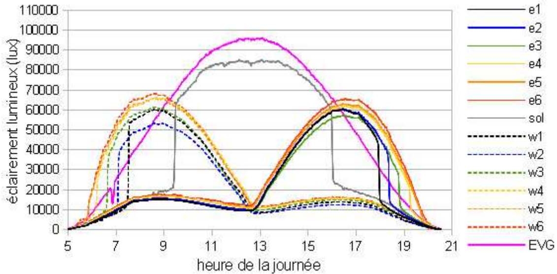
Figure IV-2 : Éclairéments lumineux mesurés sur la maquette pour H/W=0,5 avec les façades blanches le 29/06/12
