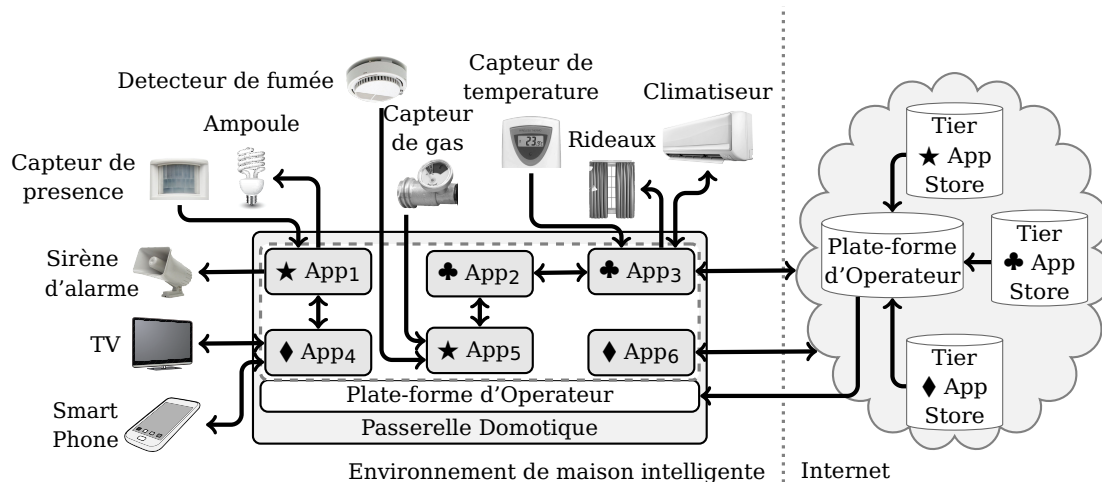
Figure 1.1: Structure domotique. Les communications entre la «Plate-forme d'Opérateur» et App1,...,App6 sont omises pour simplifier la figure.
