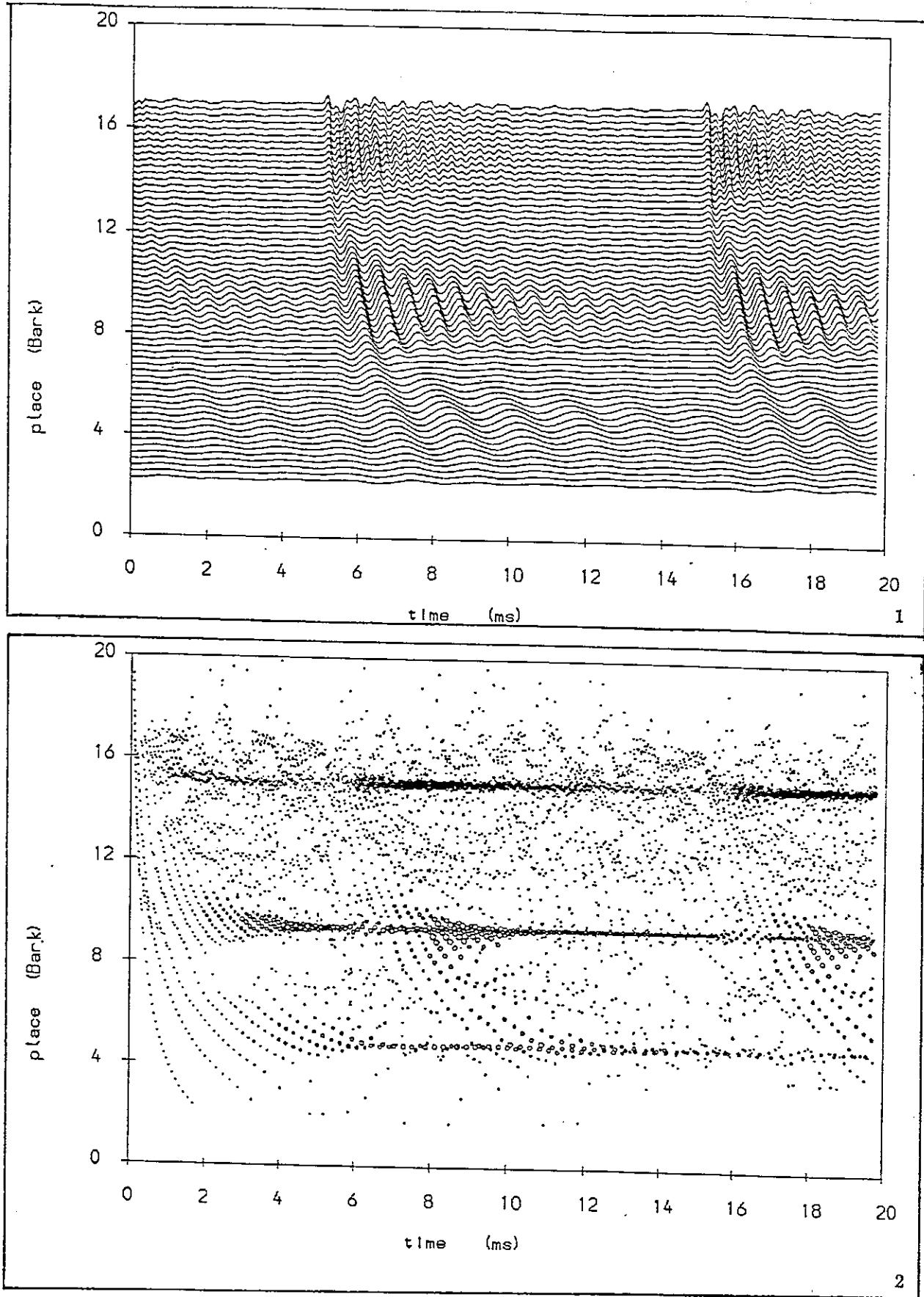
Figure 2.5: modèle de Cooke: banc de filtres et détection des fréquences, d'après Cooke, (voir texte).
