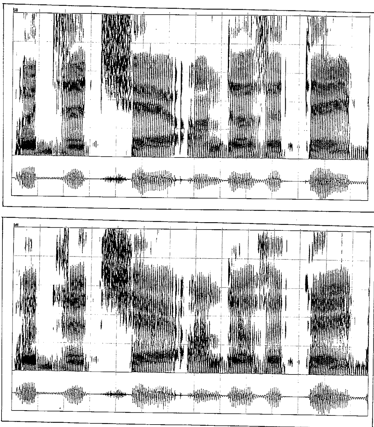
Figure 3.14: spectrogramme de "put the chair under the table", locuteur masculin, parole naturelle (haut) et synthétique (bas).
