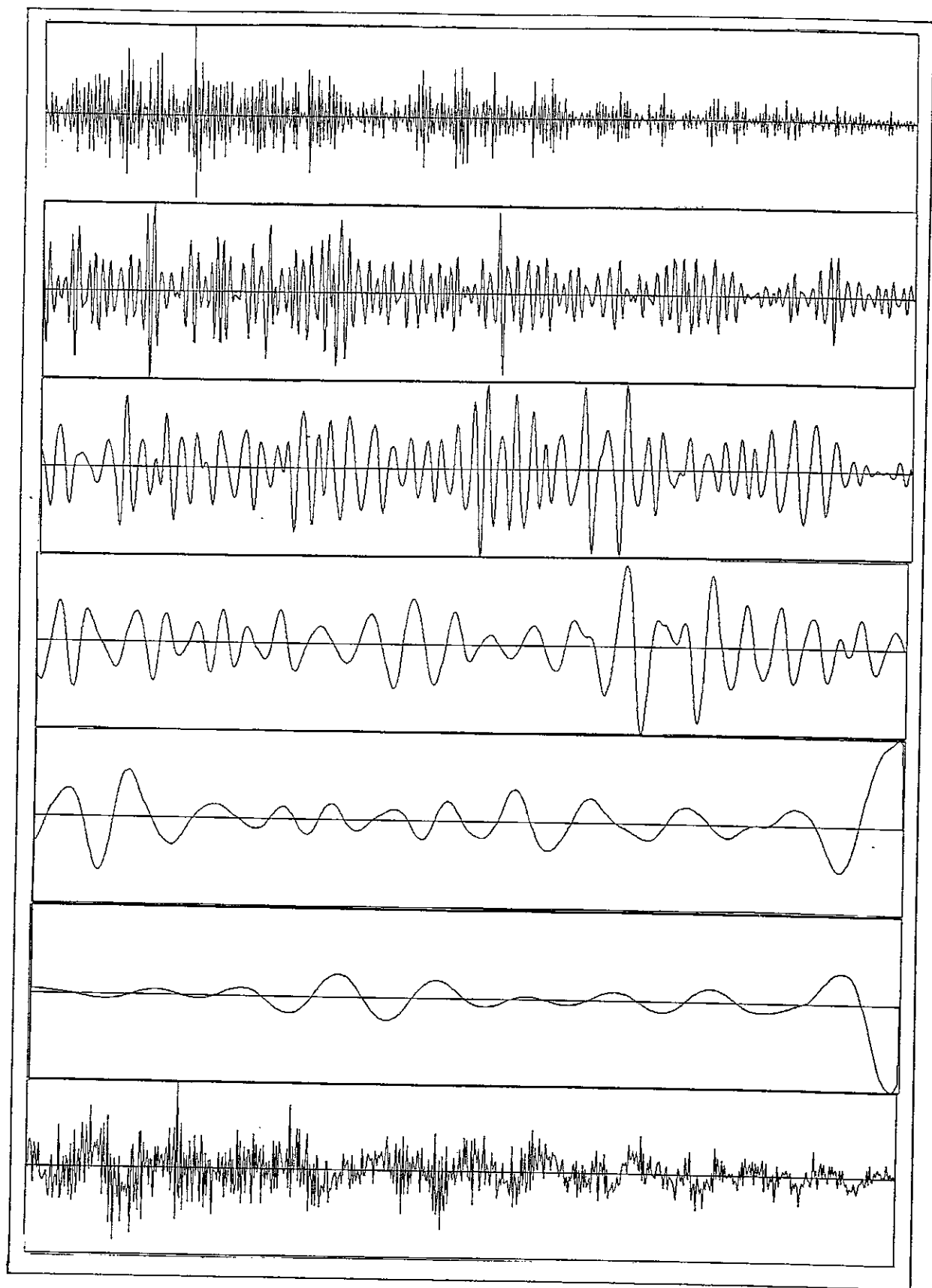
Figure 1.9: première résolution et détails additionnels d'un /s/ par transformation en ondelettes orthogonales utilisant des filtres miroir en quadrature (voir texte).
