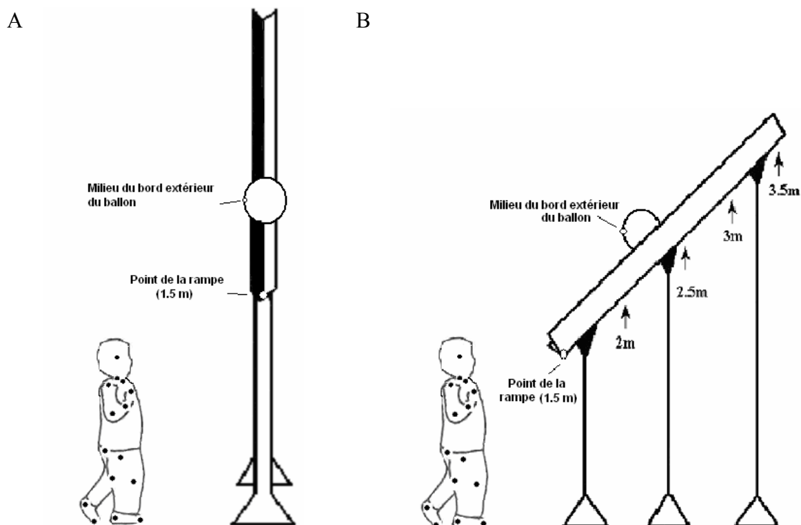
Figure 64. Points utilisés pour le pointage image par image. Figure A : Points utilisés pour le pointage image quand l'enfant est face à la rampe. Figure B : Points utilisés pour le pointage image quand l'enfant est de côté par rapport à la rampe.
