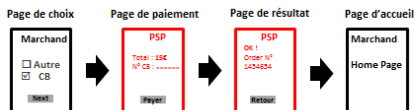
FIGURE 4.10 – Cinématique n°1 : l'E-commerçant délègue l'affichage du ticket de paiement à son prestataire de paiement bancaire
