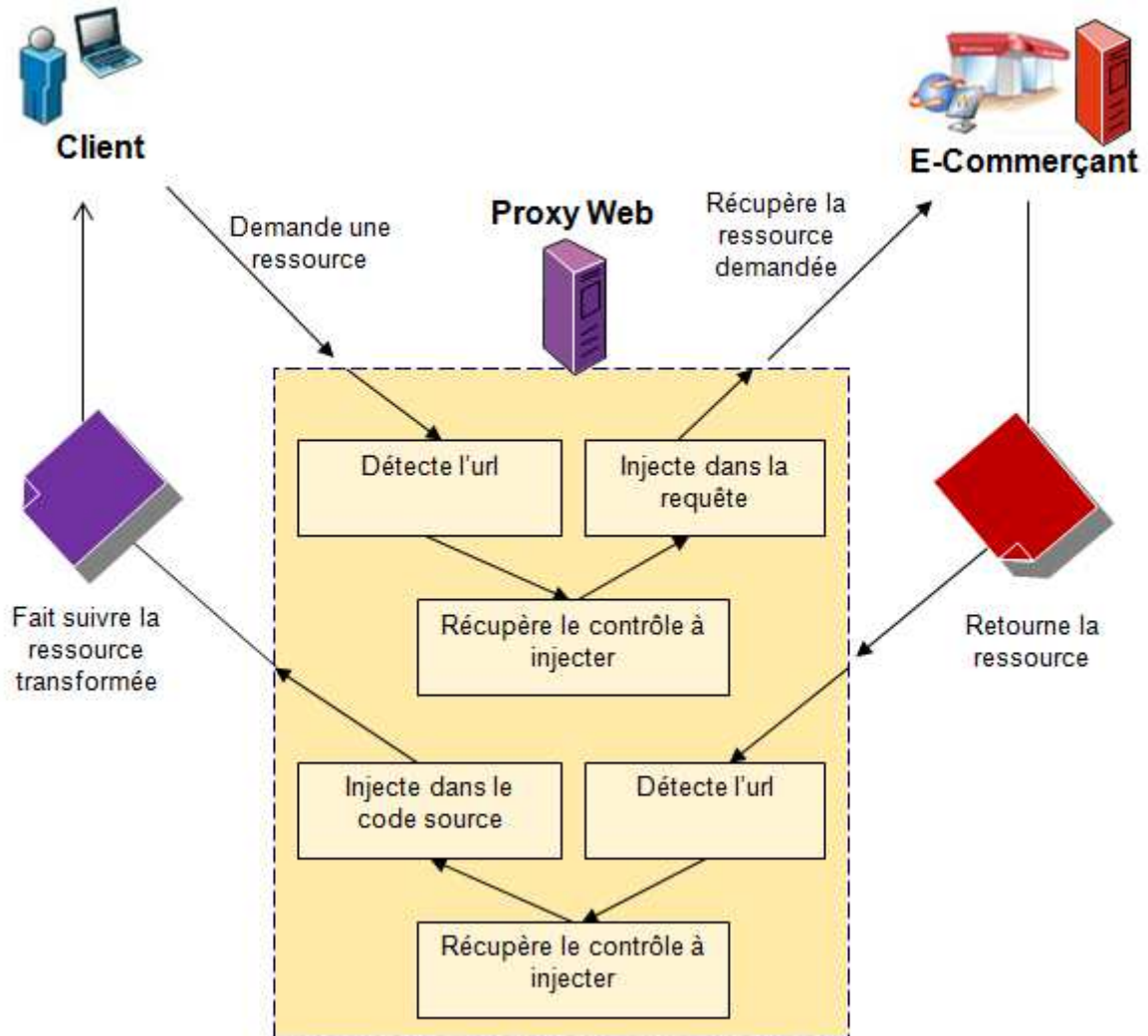
FIGURE 4.4 – Processus d'injection avec Proxy Web
