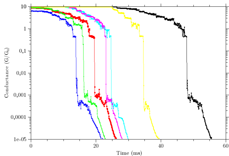
FIGURE 4.4 – Mesures de conductance réalisées dans une solution millimolaire de 4,4' bipyridine dans le toluène. Des plateaux de conductance sont mesurés entre 10^{-4} et 10^{-3} G_0
