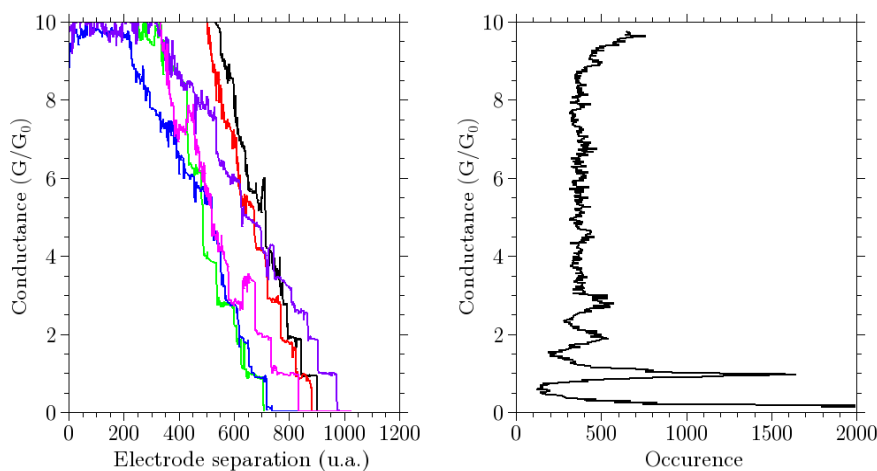
FIGURE 4.2 – Gauche : Mesures G(z) sur une constriction d'or mettant en évidence la quantification de la conductance en multiples entiers de G_0 = 2e^2/h . Mesures réalisées en STM-BJ, vitesse de retrait des électrodes 1\text{nm}\cdot\text{s}^{-1} , polarisation des électrodes 130\text{ mV} .
