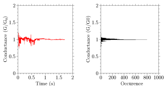
FIGURE 5.1 – Gauche : Trace G(t) enregistrée sur une constriction d'or dont on a stoppé l'étiement lorsque la conductance atteint la valeur de G_0 . A noter que la structure est stable plusieurs secondes. Des fluctuations de conductance sont observées autour d'une valeur moyenne de G .
