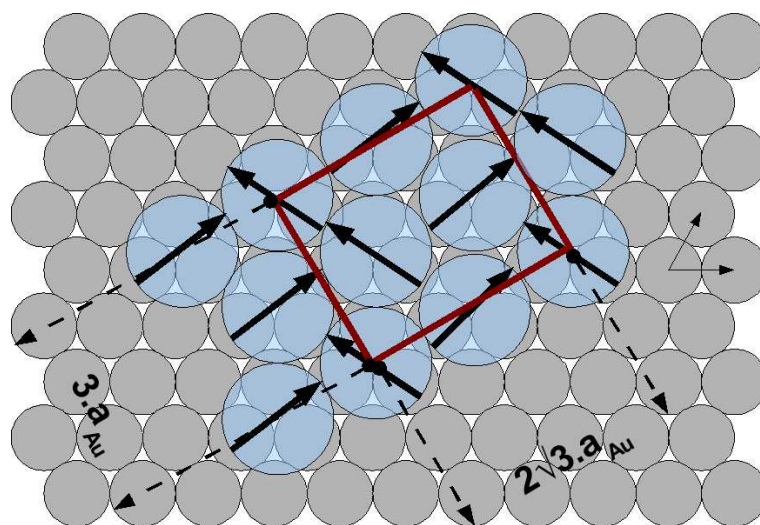
FIGURE 1.2 – Représentation schématique d’une surstructure c(4 \times 2) . La reconstruction résultante est une 3 \times 2\sqrt{3} R30^\circ relative à la surface d’Au (111) [4]. Les molécules sont toutes inclinées d’un angle de 30^\circ par rapport à la normale à la surface. Sur le schéma, des orientations possibles du plan contenant le squelette carboné des molécules sont représentés par des flèches.
