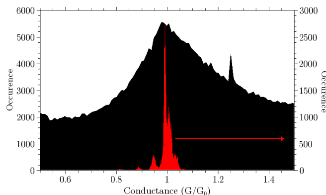
FIGURE 5.2 – Comparaison d'un histogramme de conductance cumulé sur 36600 traces G(z) (512 points par trace) et de l'historgramme d'une trace G(t) (50000 points, fréquence d'acquisition 30 kHz). Autour de G_0 la largeur à mi-hauteur du pic de l'historgramme des G(z) (en noir) est d'environ 0.4 G_0 , comparé à 0.04 G_0 pour l'historgramme de la trace G(t) (en rouge). Les fluctuations observées sur une trace G(t) , seules, ne peuvent expliquer la largeur de l'historgramme global.
