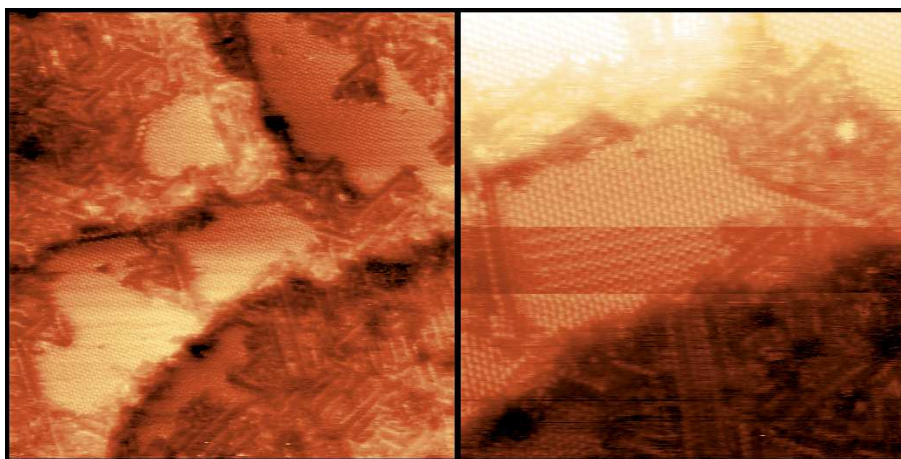
FIGURE 2.1 – Images STM d'un film d'or immergé 30 s dans une solution de décanethiol.
