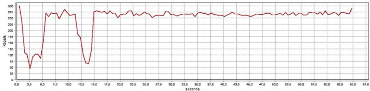
FIGURE 5.13 Débit au niveau applicatif pour le cas non streamé en utilisant ETP (CdS RT Interactive)
