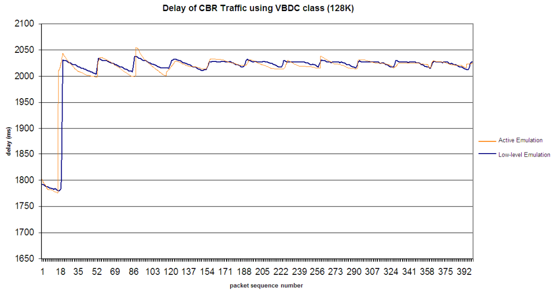
FIGURE 5.34 Evolution du délai des paquets dans le cas d'une classe VBDC à 128K
