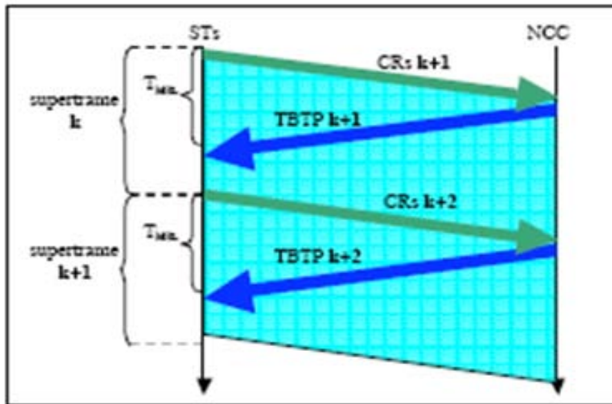
FIGURE 5.26 Principe de requête / allocation du DAMA
