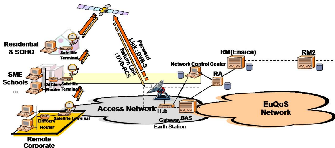
FIGURE 5.27 Liaison satellite dans le réseau EuQoS
