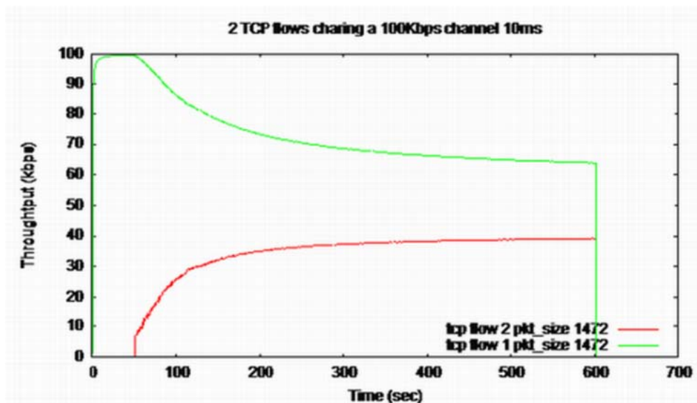
FIGURE 4.9 Deux flux TCP se partageant un canal
