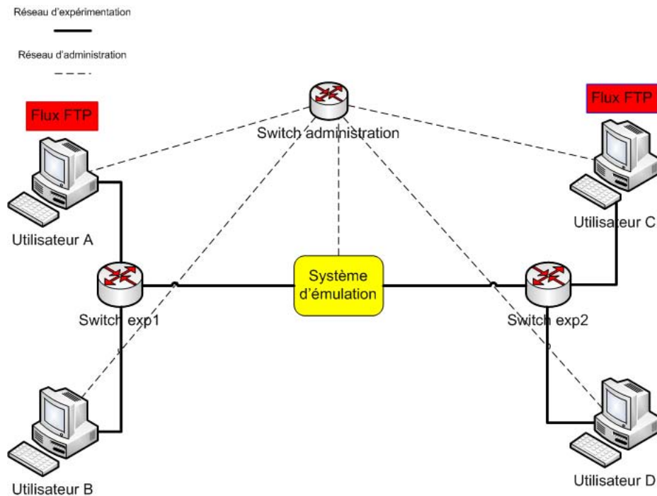
FIGURE 5.32 Plate-forme d'expérimentation
