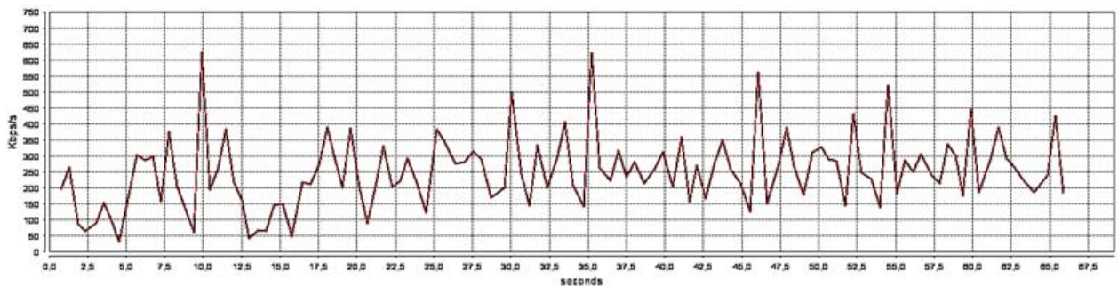
FIGURE 5.15 Débit au niveau applicatif pour le cas non streamé en utilisant ETP (CdS Standard)
