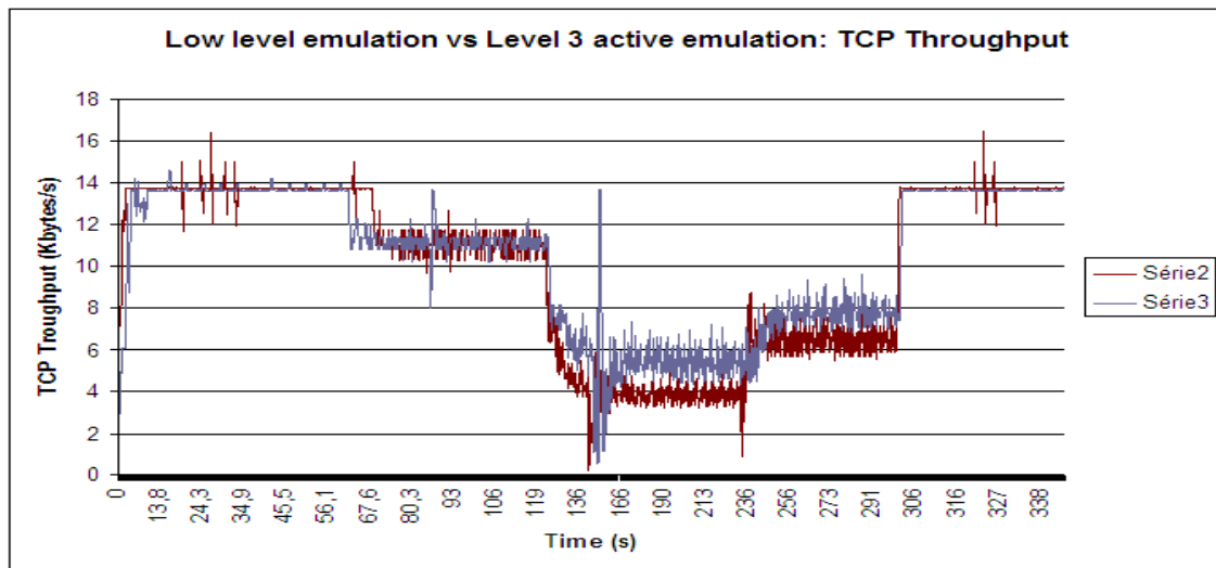
FIGURE 5.37 Comparaison des résultats obtenus par émulation de niveau 2 et 3 pour le cas du débit du flux TCP
