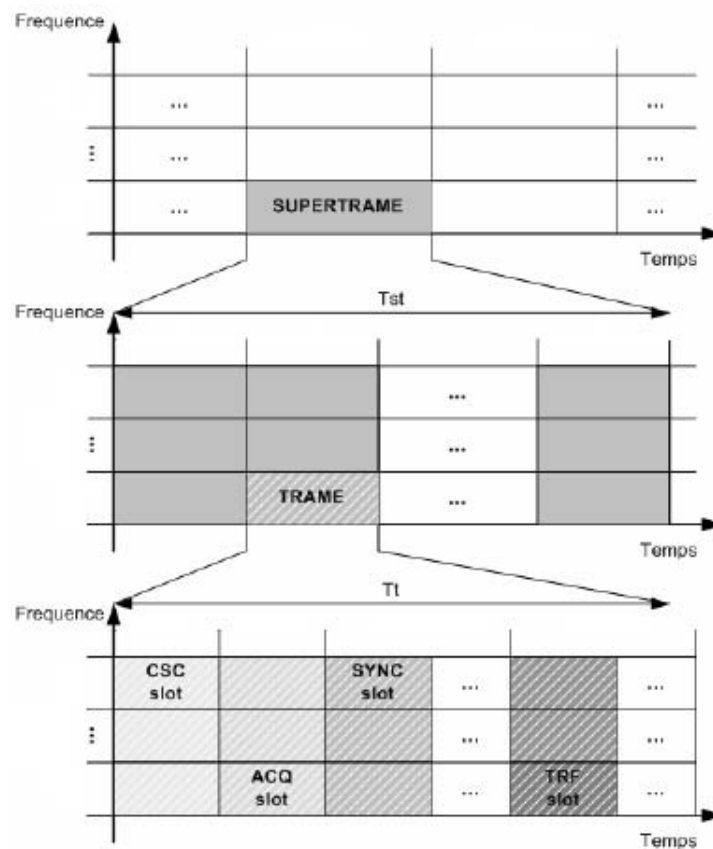
FIGURE 5.25 Format d'une supertrame DVB-RCS
