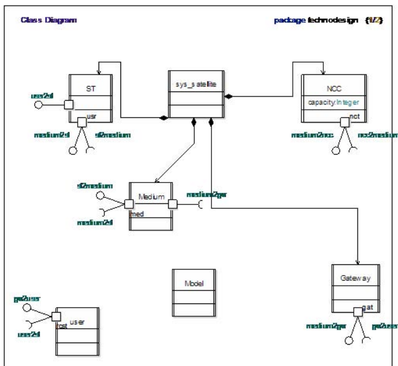
FIGURE 3.3 Modèle de technologie d'une liaison satellite
