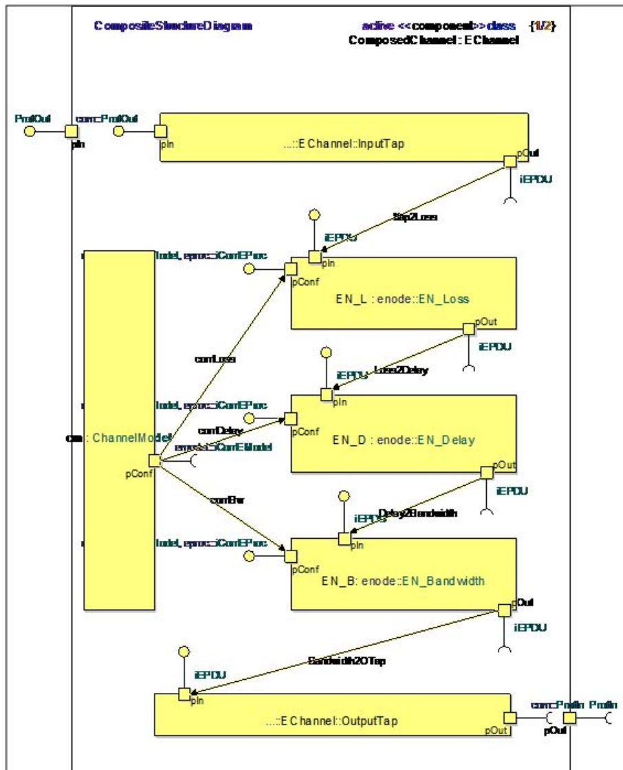
FIGURE 3.6 Composite Structure Diagram du canal d'émulation
