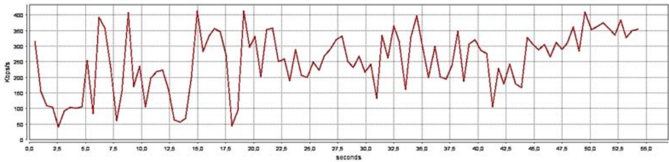
FIGURE 5.9 Débit au niveau applicatif pour le cas non streamé en utilisant UDP
