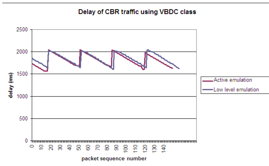
FIGURE 5.33 Délai des paquets en VBDC
