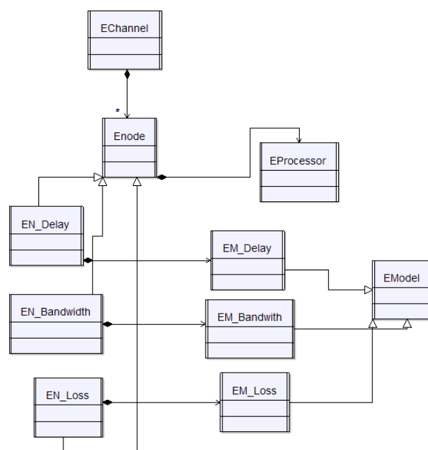
FIGURE 3.5 Diagramme de classes du canal d'émulation
