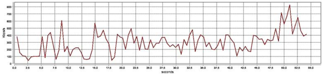
FIGURE 5.18 Débit au niveau applicatif pour le cas streamé en utilisant UDP
