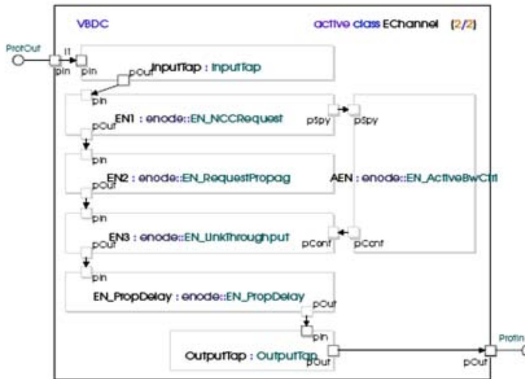
FIGURE 5.31 Modélisation du VBDC
