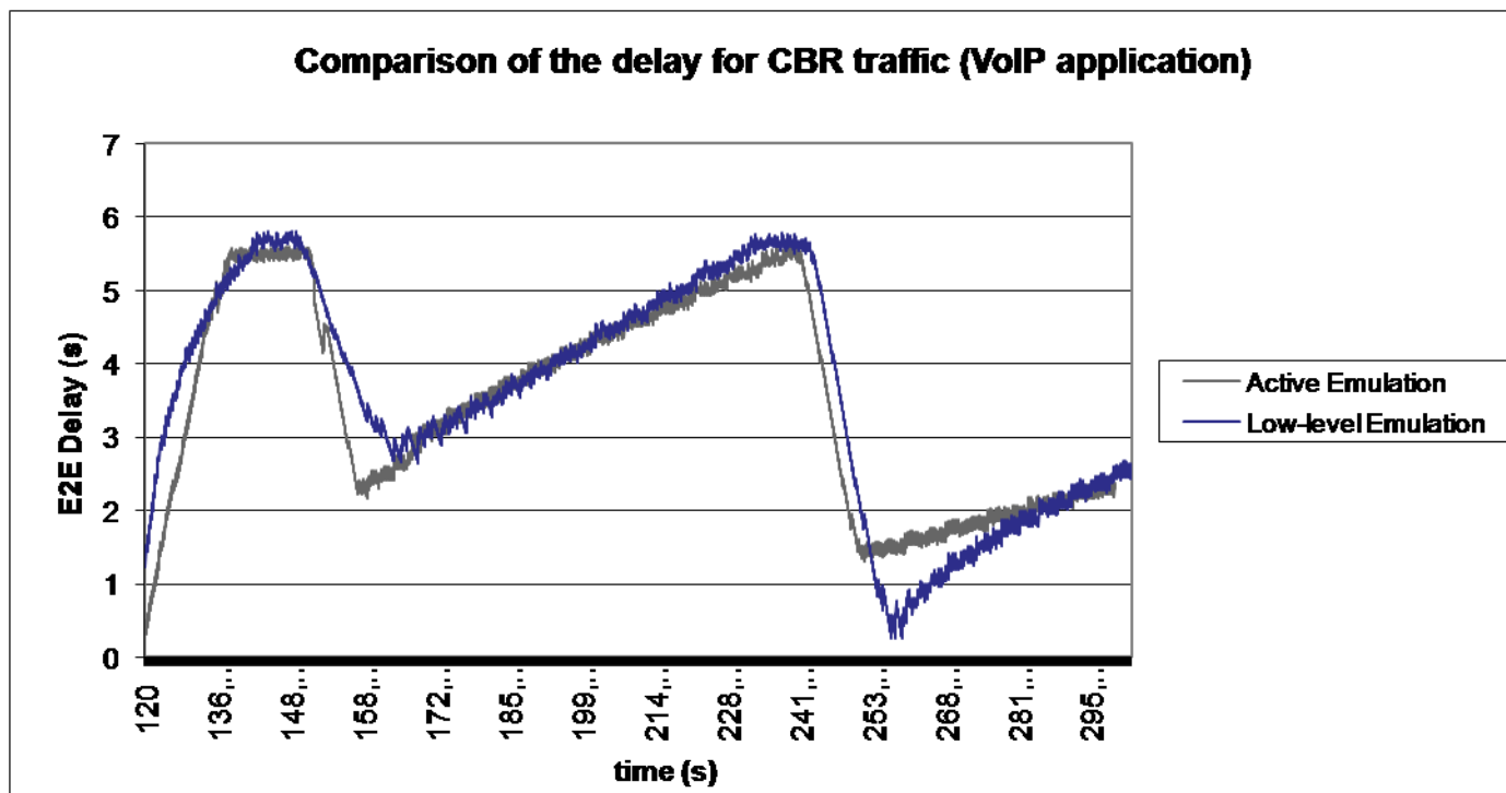
FIGURE 5.38 Evolution du délai de bout en bout du trafic CBR dans le cadre d'application de VoIP
