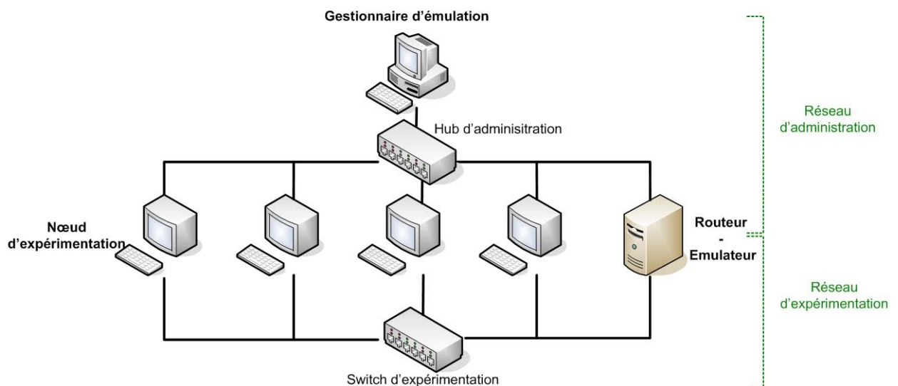
FIGURE 5.3 Architecture de la plate-forme d'émulation NINE
