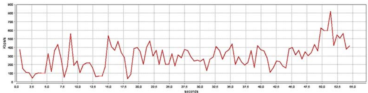
FIGURE 5.21 Taux de pertes pour une application streamée utilisant TCP
