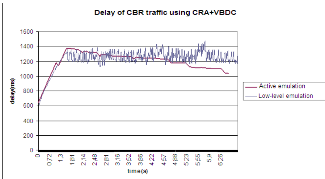
FIGURE 5.34 Evolution du délai des paquets dans le cas d'une classe VBDC à 128K
