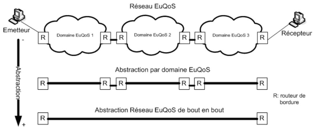
FIGURE 5.5 Abstraction réseau EuQoS
