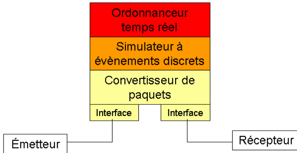
FIGURE 2.7 Architecture émulateur par simulation temps réel
