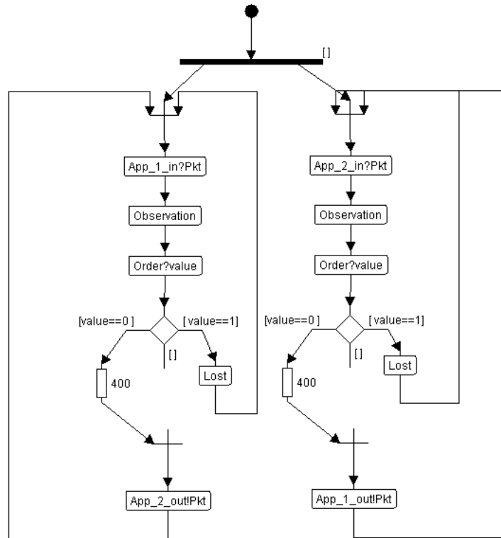
FIGURE 3.9 Description du comportement du processeur
