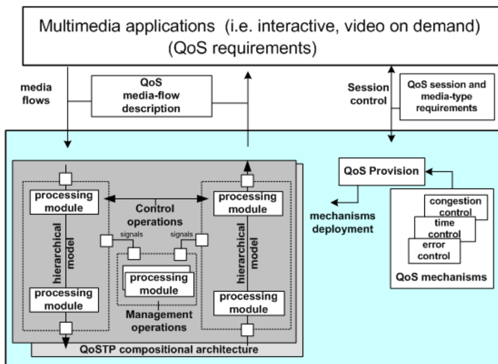
FIGURE 5.2 Vision globale des mécanismes du protocole ETP
