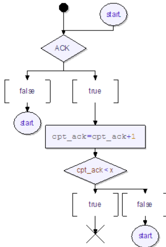
FIGURE 4.6 Exemple de machine à état
