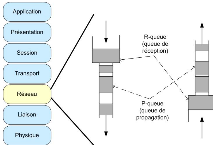
FIGURE 2.5 Fonctionnement de Dummynet
