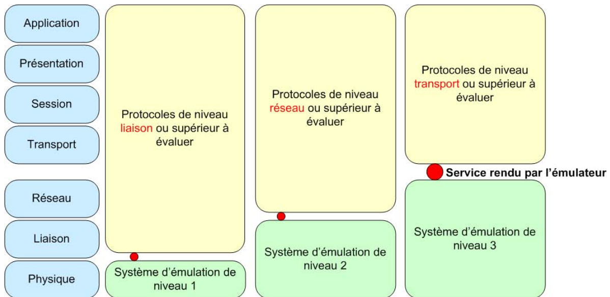
FIGURE 2.2 Différents niveaux d'émulation réseau
