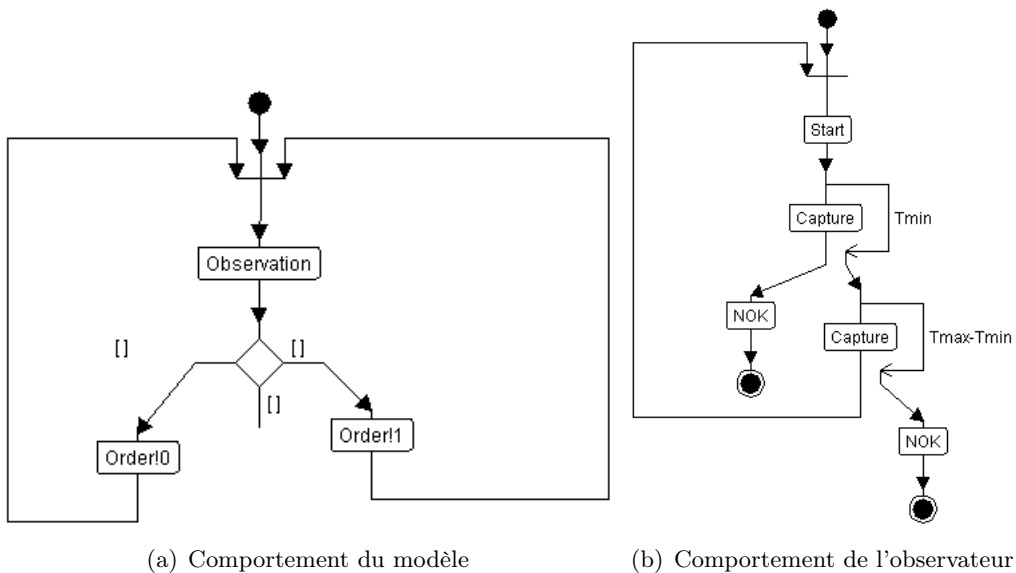
FIGURE 3.10 Comportements du modèle et de l'observateur
