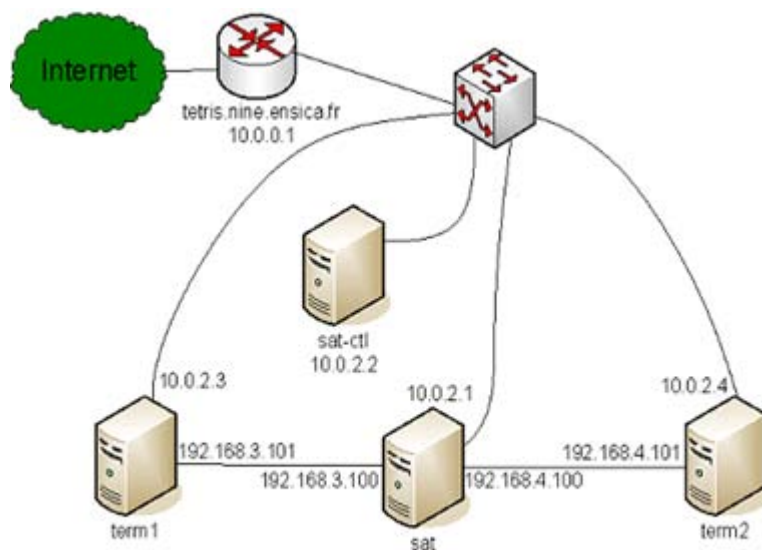
FIGURE 5.4 Architecture de la plate-forme d'émulation
