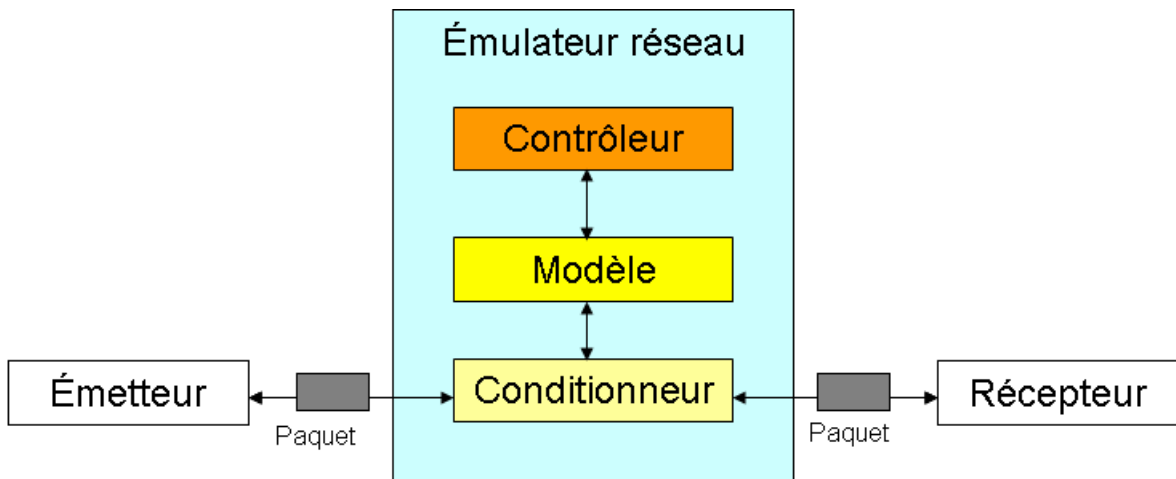
FIGURE 3.1 Architecture classique d'un émulateur
