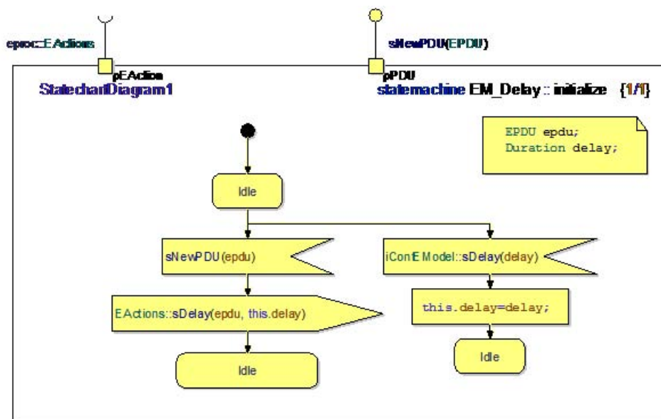
FIGURE 3.7 Exemple de modèle d'émulation de délai
