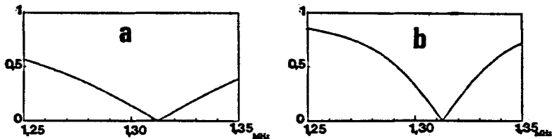
Figure 7: Module du coefficient de réflexion en fonction de la fréquence, mode S_1 . a: Coefficient de réflexion exact. b: Coefficient de réflexion obtenu par série de Debye pour N=10 .
