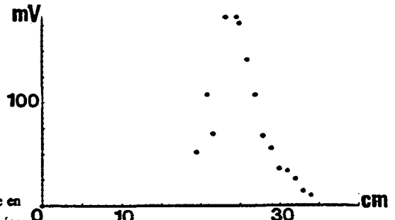
Figure 4: Evolution de l'amplitude d'un écho de forme losange en fonction de la distance par rapport à l'extrémité de la plaque. Mode incident S_3 , réception sous l'angle de réémission du mode A_1 , fd=6,5 kHz m.
