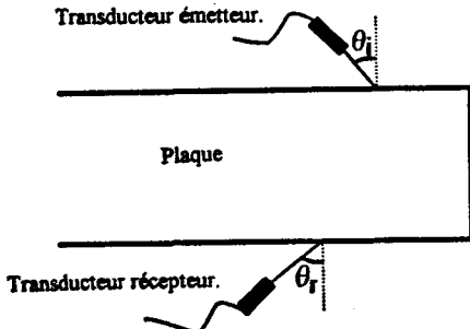
Figure 1: Géométrie de l'expérience.
