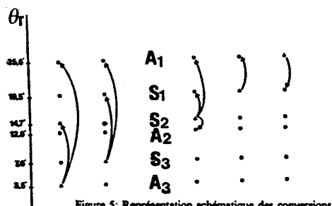
Figure 5: Représentation schématique des conversions observées à fd=6,5 kHz m. Les flèches partent du mode incident et arrivent sur les modes convertis.
