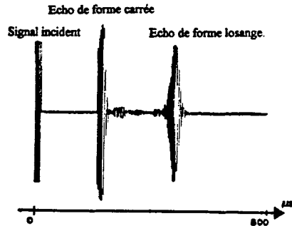
Figure 2: Exemple de réception d'un écho de forme carrée et d'un écho de forme losange. Mode incident S_3 , fd=6,5 kHz m.
