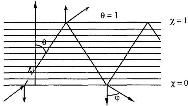
Fig. 4. — Le trajet des rayons dans le mur.
