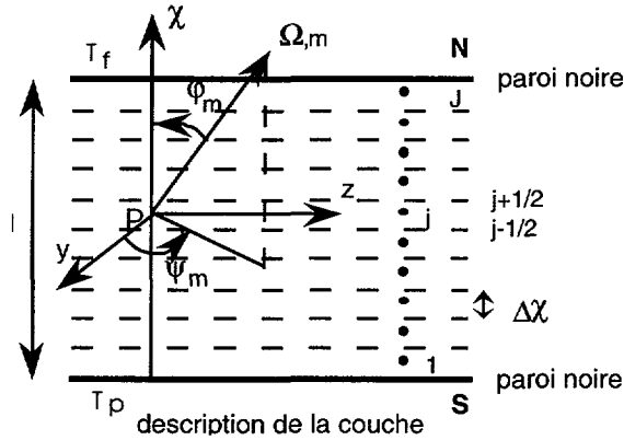
Fig. 3. — Système d'axes de la méthode des ordonnées discrètes.
