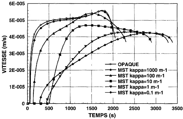
Fig. 8. — Évolution de la vitesse de fusion d'un mur plan gris de 10 cm en fonction du temps pour différents coefficients d'absorption.
