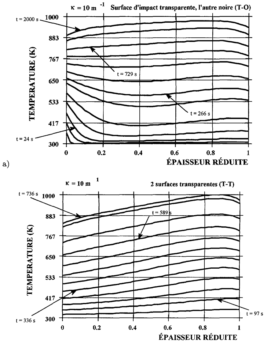
Fig. 9. — Profils de température dans le mur de MST gris de coefficient d'absorption 10 \text{ m}^{-1} à différents instants, a) surface d'impact transparente, surface fixe opaque noire, b) les deux interfaces transparentes.
