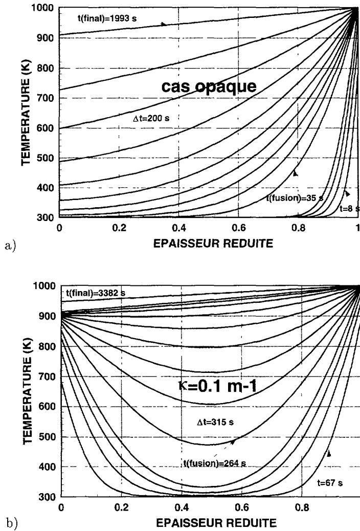
Fig. 5. — Profils de température dans le mur à parois noires à différents instants, a) cas opaque. b) mur gris de coefficient d'absorption 0,1 \text{ m}^{-1}
