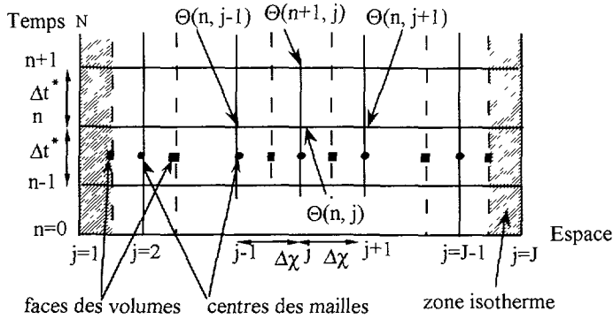
Fig. 2. — Maillage spatio-temporel du mur.
