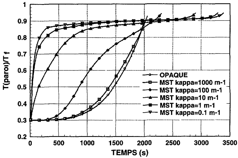
Fig. 6. — Évolution en fonction du temps de la température d'une paroi fixe noire d'un mur plan de 10 cm pour différents coefficients d'absorption.
