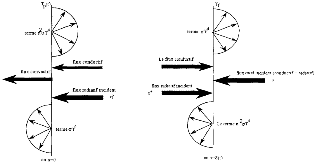
Fig. 1. — Les conditions aux limites thermiques en flux du mur plan de MST. [Thermal boundary conditions of the plane STM wall.]
