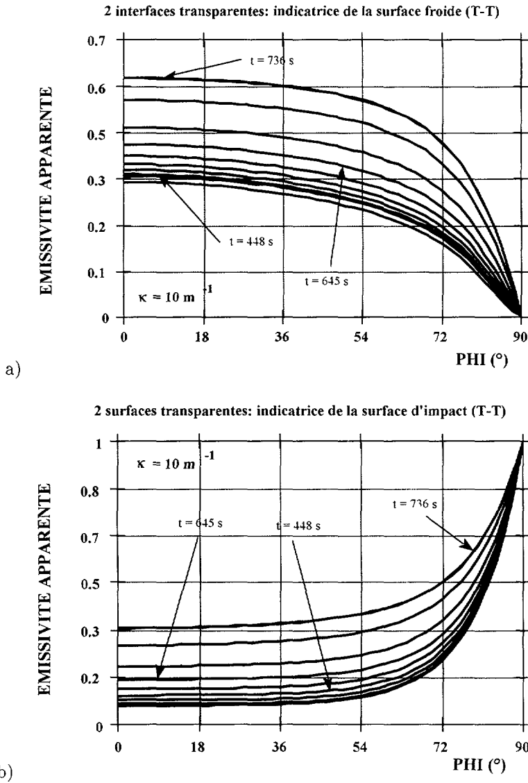
Fig. 10. — Émissivité apparente d'un mur plan de coefficient d'absorption 10 \text{ m}^{-1} avec ses deux frontières transparentes, a) pour la surface froide, b) pour la surface d'impact.
