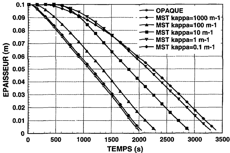
Fig. 7. — Évolution en fonction du temps de l'épaisseur d'un mur plan gris de 10 cm pour différents coefficients d'absorption.
