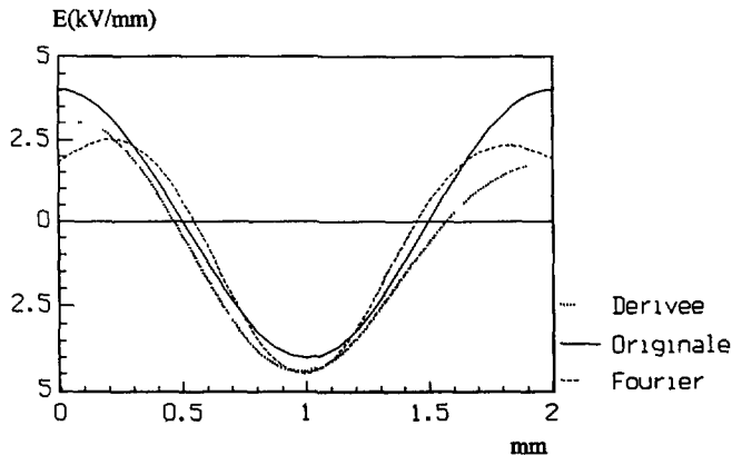
Fig. 1. — Champ électrique donné, resimulé à partir de la méthode des dérivations et par séries de Fourier.
