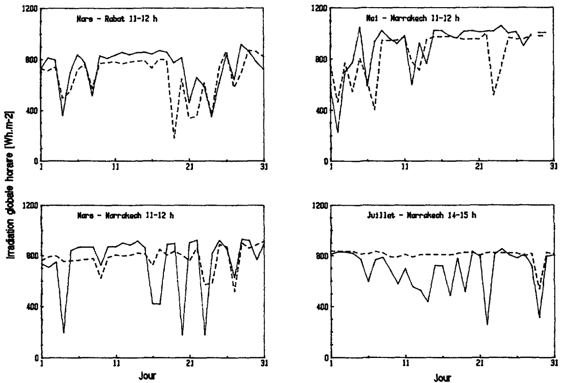
Fig. 4. — Variations des irradiances globales horaires mesurées au sol et estimées à partir des données satellitaires pour quelques mois. (—) au sol ; (----) satellite.
