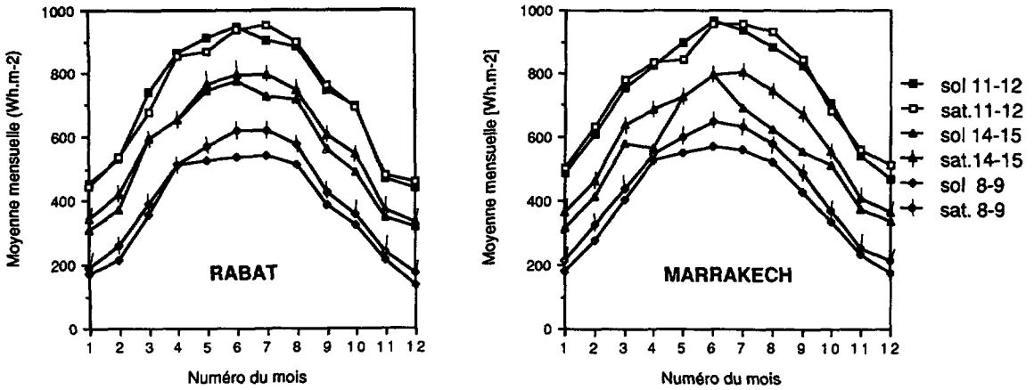
Fig. 3. — Moyennes mensuelles des irradiances globales horaires mesurées au sol et déduites des mesures satellitaires.
