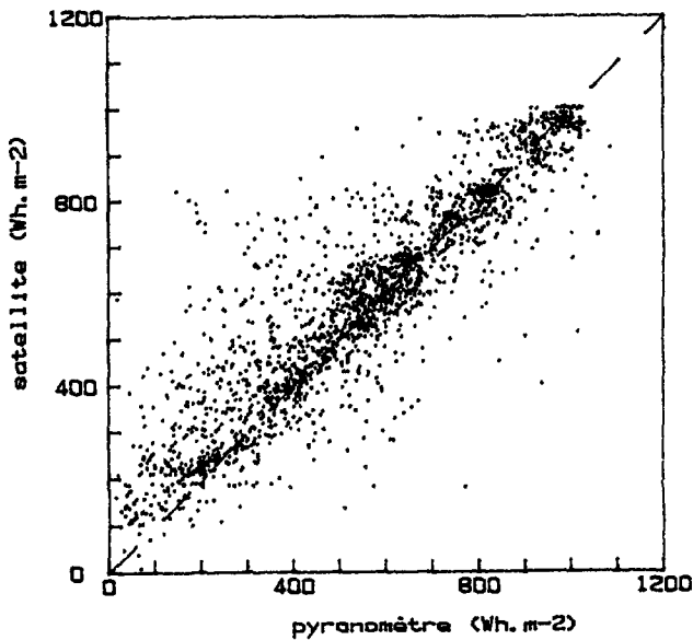
Fig. 1. — Comparaison des irradiances globales horaires mesurées au sol et estimées à partir des données satellitaires.
