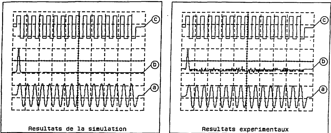
Fig. 10. — Filtre à 12 coefficients en 16 cellules.
