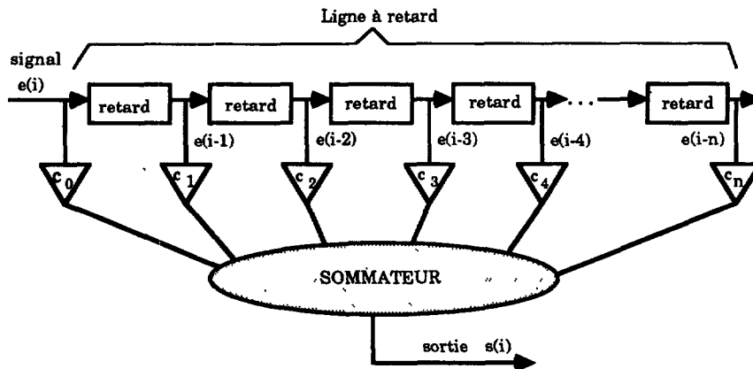
Fig. 1. — Filtre transversal.
