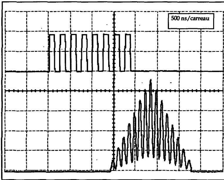
Figs. 8 et 9. — Autoconvolution de trains d'impulsions rectangulaires.
