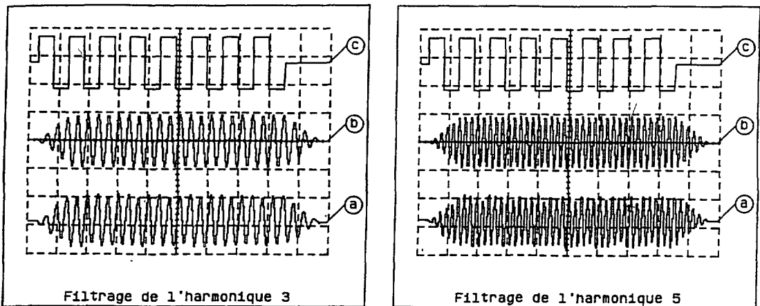
Fig. 11. — Filtrage des harmoniques d'un carré à 250 KHz.
