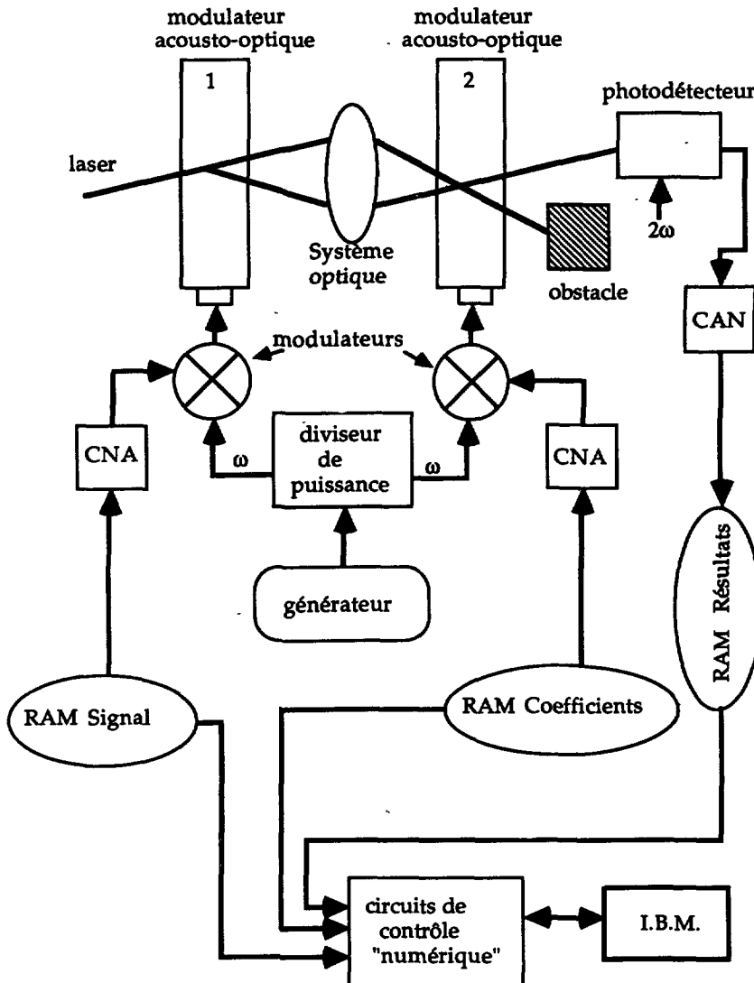
Fig. 7. — Schéma de principe de la manipulation.
