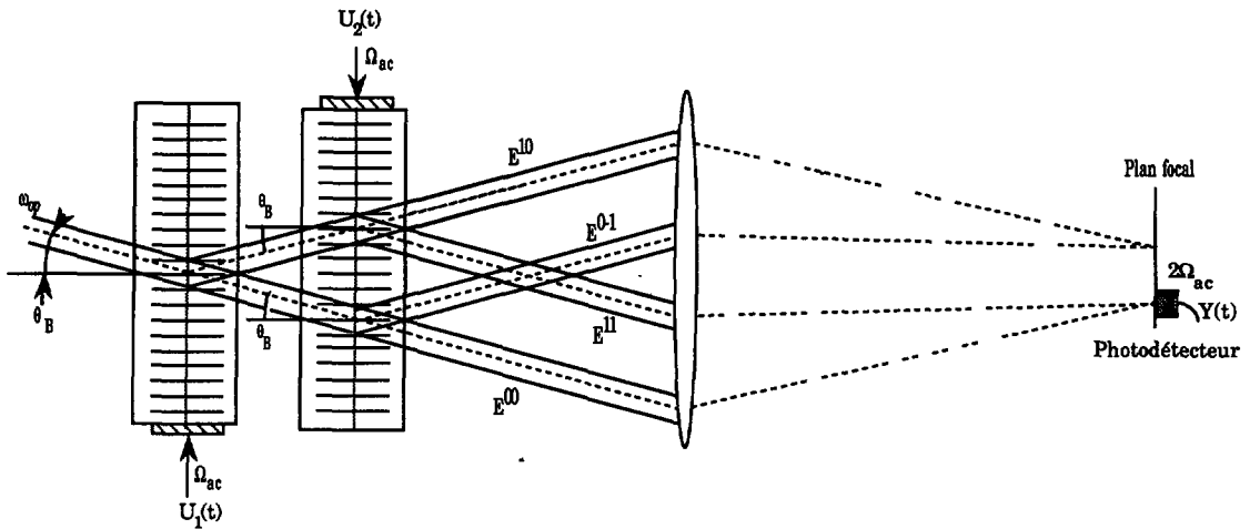
Fig. 4. — Convoluteur acousto-optique.
