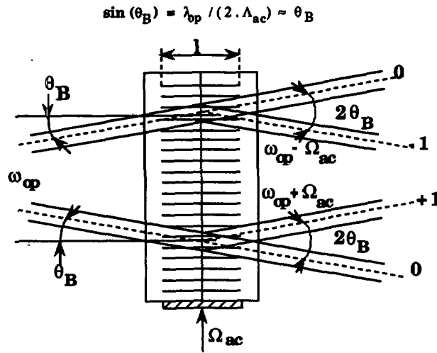
Fig. 3. — Interaction acousto-optique en régime de Bragg.
