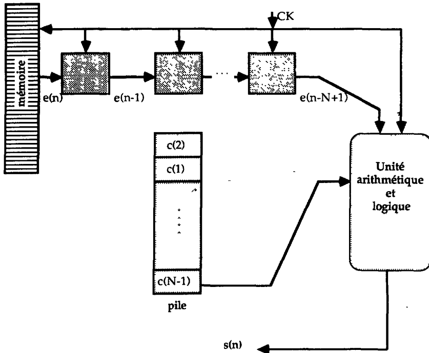
Fig. 2. — Principe d'un CTS.
