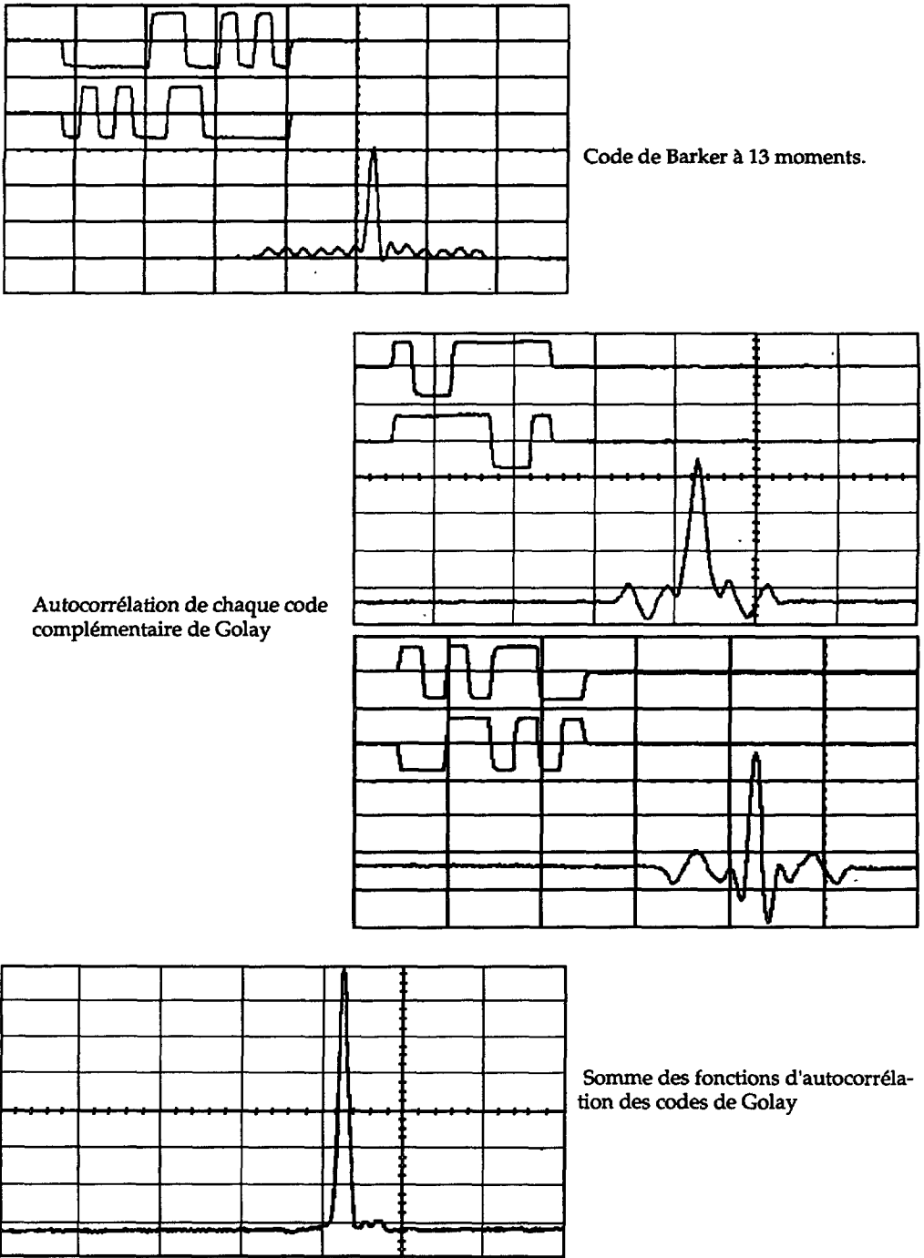
Fig. 12. — Fonction d'autocorrélation des codes de Barker et Golay.
