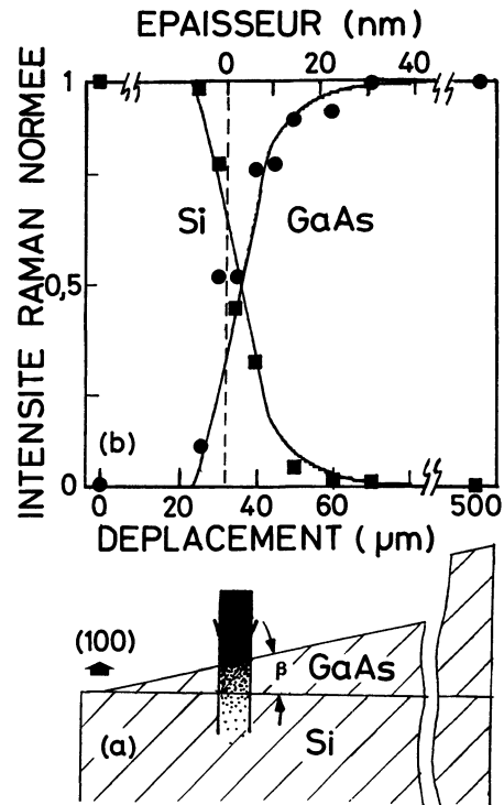
Fig. 5. — a) Coupe longitudinale de l'échantillon biseauté montrant la géométrie de diffusion. b) Variation des intensités Raman normalisées associées au Si et au GaAs en fonction du déplacement sur le biseau. L'épaisseur de la couche de GaAs est aussi indiquée.
