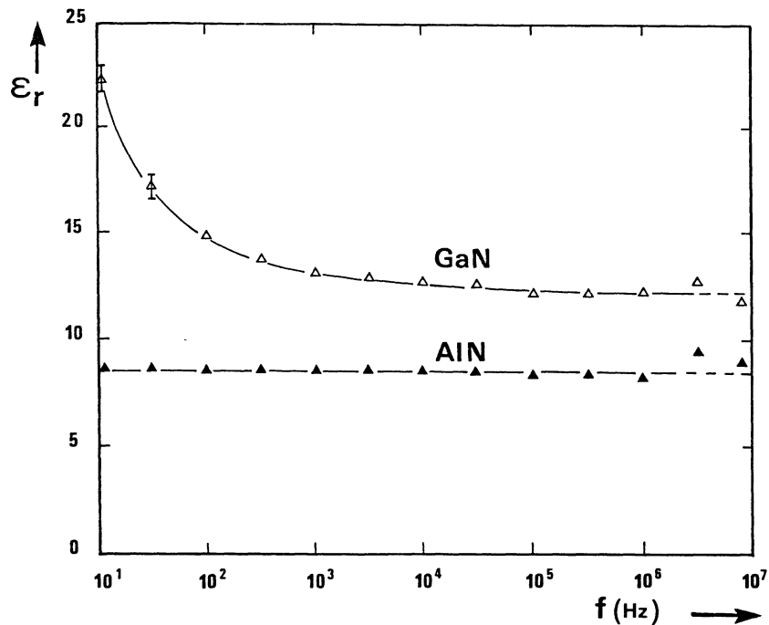
Fig. 2. — Permittivité diélectrique en fonction de la fréquence, pour des couches minces de GaN et AlN (avec E//c ).
