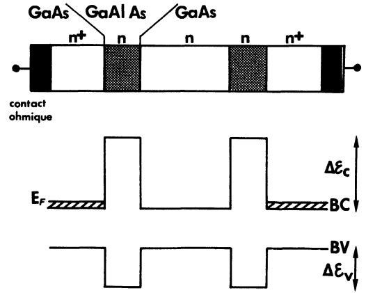
Fig. 2. — Structure schématisée de la double barrière.
