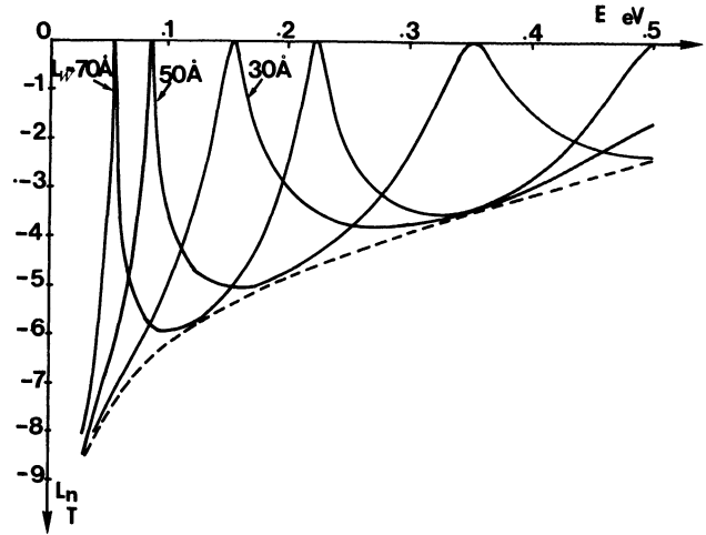
Fig. 7. — Energie de résonance en fonction de la largeur de puits quantique.
