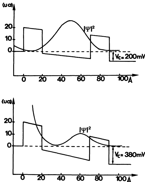
Fig. 6b. — Fonction d'onde pour des tensions de polarisation proche de la résonance et hors résonance.
