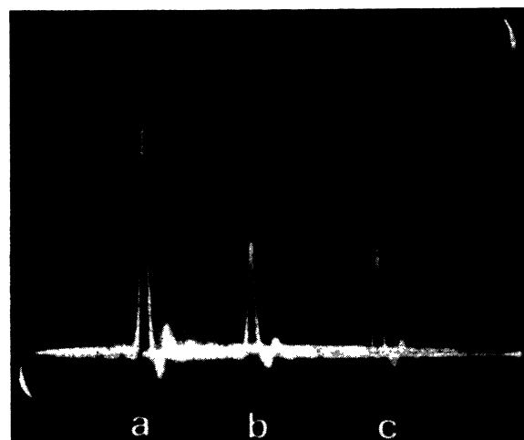
Fig. 16. — Transfert d'énergie par couplage d'ondes entre deux impulsions de durée 3 ns : faisceau sonde seul (a), faisceau sonde en présence de la pompe lors d'un tir unique (b), après plusieurs tirs (c).
