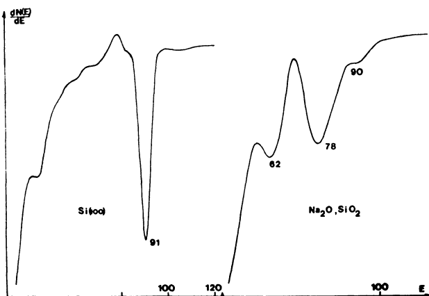
FIG. 10. — Spectre Auger du silicium et d'un verre \text{Na}_2\text{O} , \text{SiO}_2 .
