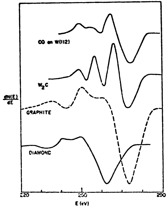
FIG. 11. — Spectre Auger du carbone dans différents composés.
