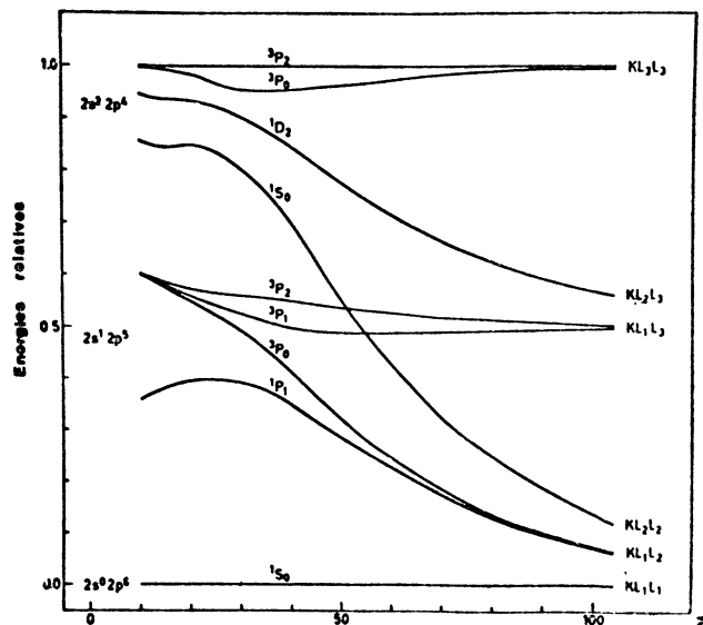
FIG. 3. — Energie relative des pics Auger KLL en fonction du numéro atomique Z .
