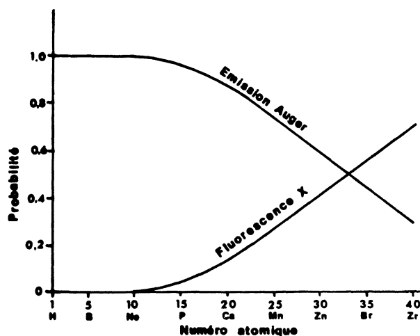
FIG. 1. — Rendement de l'émission Auger et de la fluorescence X en fonction du numéro atomique Z .
