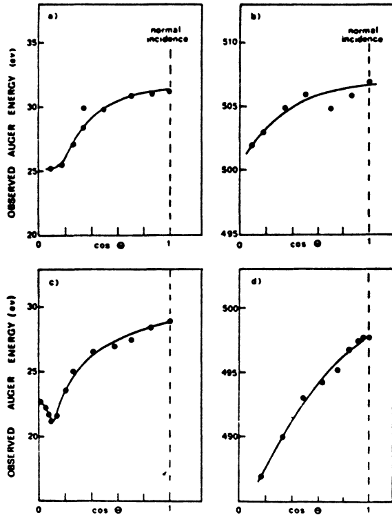
FIG. 12. — Analyse Auger du magnésium oxydé et de l'oxyde de magnésium : variation de la position du pic Auger avec l'angle d'incidence : a) Pic du magnésium dans le magnésium oxydé, b) Pic de l'oxygène dans le magnésium oxydé, c) Pic du magnésium dans la magnésie, d) Pic de l'oxygène dans la magnésie.
