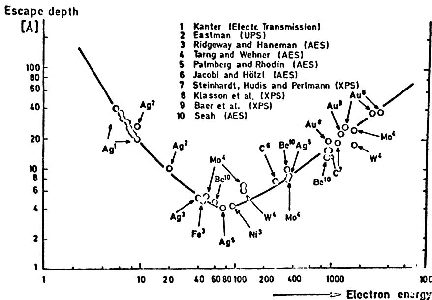
FIG. 13. — Variation du libre parcours moyen des électrons en fonction de l'énergie.
