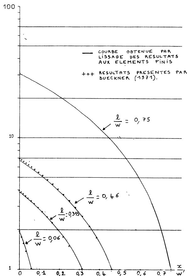
FIG. 8. — Fonction m\left(\frac{x}{W}, \frac{l}{W}\right) pour la bande infinie.
