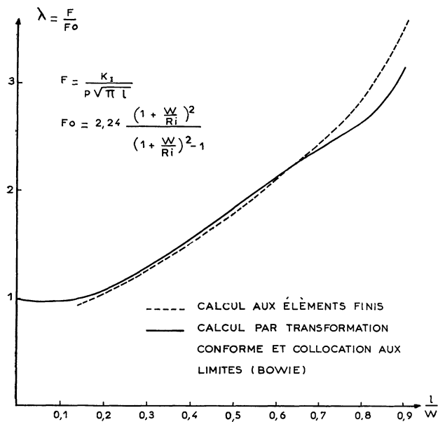
FIG. 9. — Cylindre infini avec fissure axiale soumis à une pression intérieure p pour R_i/W = 2 .
