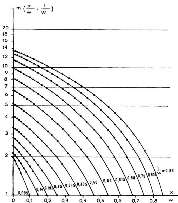
FIG. 10. — Fissure longitudinale \frac{R}{W} = 5 . Fonction m(\frac{x}{W}, \frac{l}{W})
