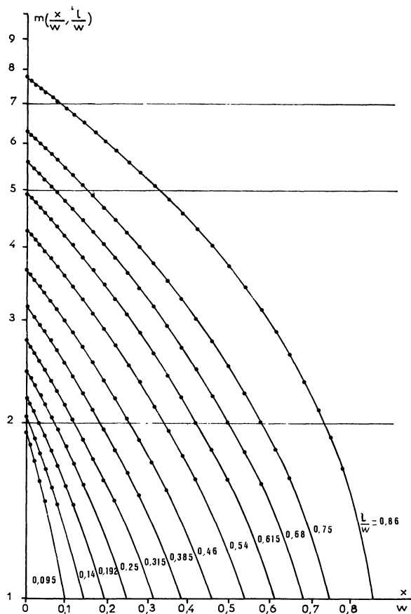
FIG. 11. — Fissure circconférentielle \frac{R}{W} = 5 . Fonction m(\frac{x}{W}, \frac{l}{W})
