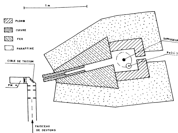
FIG. 1. — Schéma du dispositif expérimental utilisé pour l'étude de réactions (n, n'\gamma) .
