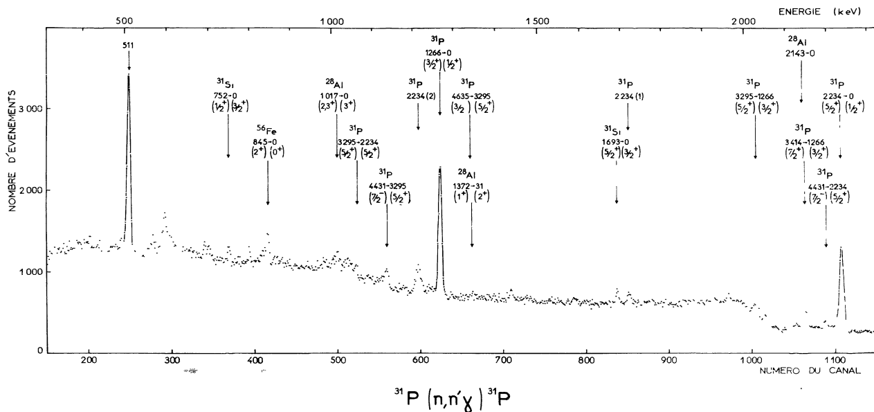
FIG. 2. — Spectre du rayonnement \gamma émis à 90^\circ par un diffuseur de ^{31}\text{P} bombardé par des neutrons de 14,5 MeV.
