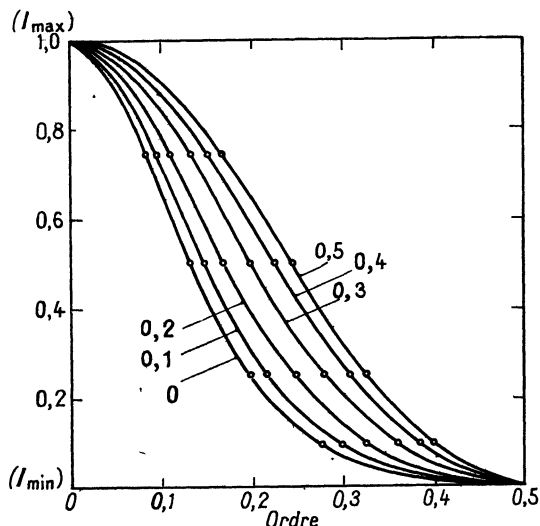
FIG. 3 a. — Profils corrigés calculés pour \rho = 0,48 et \mu = 0 ; 0,1 ; 0,2 ; 0,3 ; 0,4 ; 0,5 , élargis par un trou d'exploration de 0,175 ordre de rayon.
