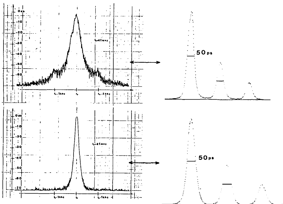
Fig.1 : Histogrammes d'impulsions lumineuses uniques ( \lambda = 532 \text{ nm} ). Courbes de variations des durées et des intensités crêtes de ces impulsions au cours du temps
