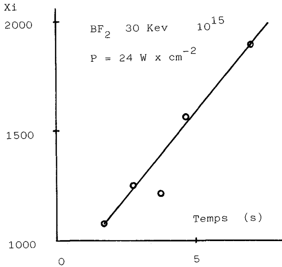
Fig. 3 - Profondeur de jonction en fonction du temps de recuit
