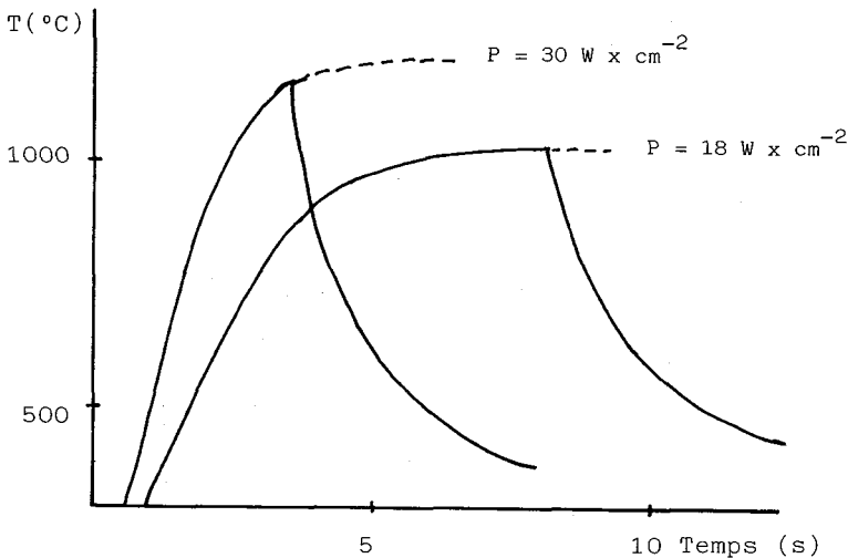
Fig. 1 - Température en fonction du temps
