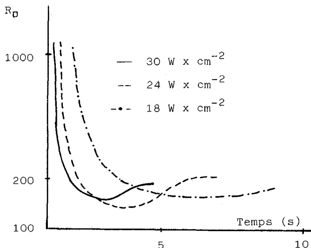
Fig. 2 - R_D en fonction du temps de recuit
