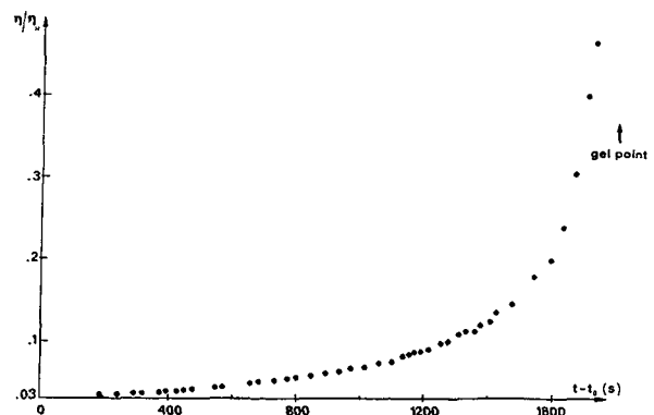
Fig. 4 : Diagramme viscosité temps pour un mélange styrène divinyl-benzène en cours de polymérisation : près du point de gel, la viscosité monte de plus d'une décade. La viscosité de normalisation \eta_R vaut 30 poises. (Enregistrement M. Adam, M. Delsanti).
