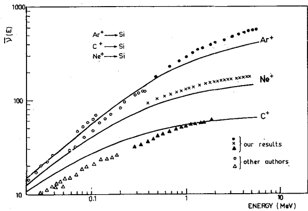
FIG. 23. — Energie perdue en collisions nucléaires dans le silicium par des ions Ar + , Ne + , C + dans un grand domaine énergétique.
