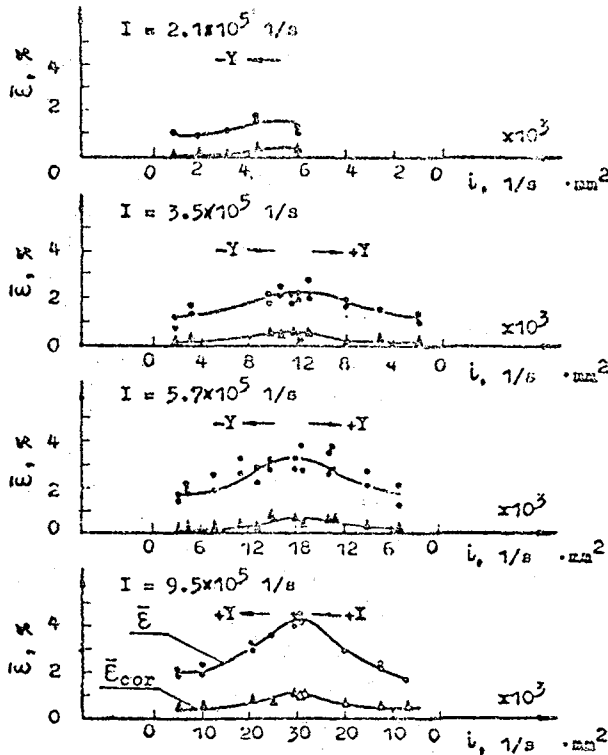
FIG. 1. — Inefficacités \epsilon et inefficacité corrélée de 2 chambres \epsilon mesurée le long d'un fil (intensité i /millimètre de fil) pour différents taux de comptage intégré ( I ) (Réf. [5]).
