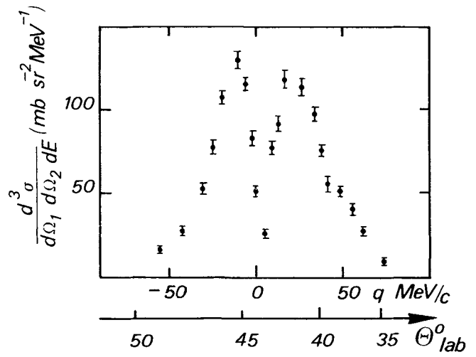
FIG. 3. — {}^6\text{Li}(\alpha, 2\alpha)d à 42,8 MeV.
