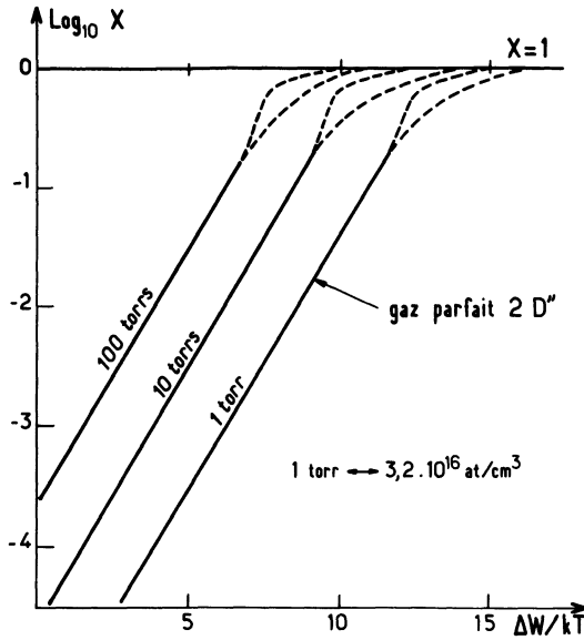
Fig. 11b. — Taux de remplissage d'une monocouche X en fonction de \Delta W/kT , pour un modèle de gaz bidimensionnel adsorbé. A haute température ( X \ll 1 ), X est donné par la formule simple (déduite de l'expression (2)) :
