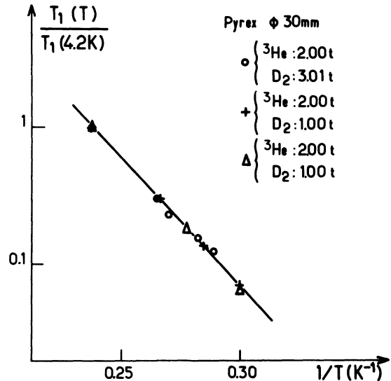
Fig. 9. — Relaxation sur D_2 solide : variation de T_1(T)/T_1(4,2K) en fonction de 1/T . Comme sur la figure 6, la droite tracée correspond à \alpha = 0 . Sa pente est q \Delta W = 42 \pm 2 K. L'incertitude sur \alpha et l'imprécision expérimentale conduisent à q \Delta W = 40 \pm 5 K.
