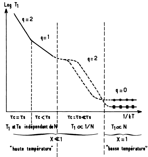
Fig. 12. — Comportement de Log T_1 en fonction de 1/T lorsqu'on peut observer un régime intermédiaire de self-diffusion des atomes adsorbés dans les gradients de champ créés par la paroi.
