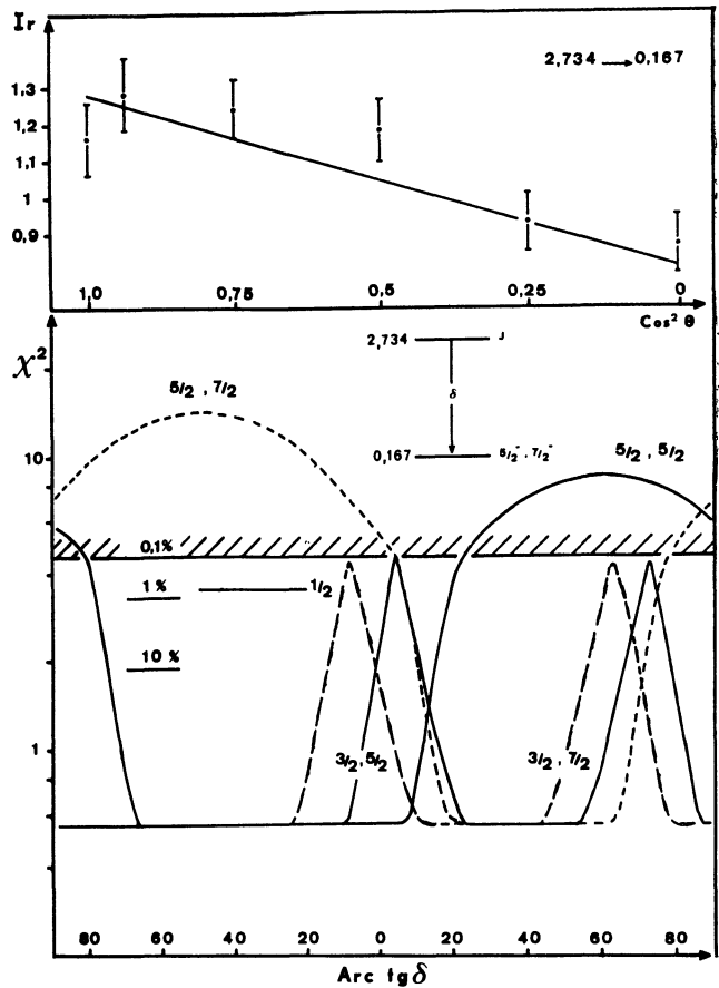
FIG. 6. — Corrélation angulaire et analyse en \chi^2 de la transition (2,734 \rightarrow 0,167 MeV) du niveau à 2,734 MeV de ^{41}\text{A} .
