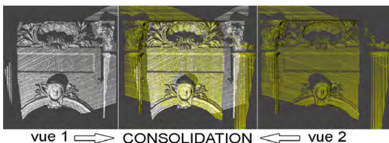
Figure 17 - Exemple de consolidation de deux nuages (Fuchs, 2006).
