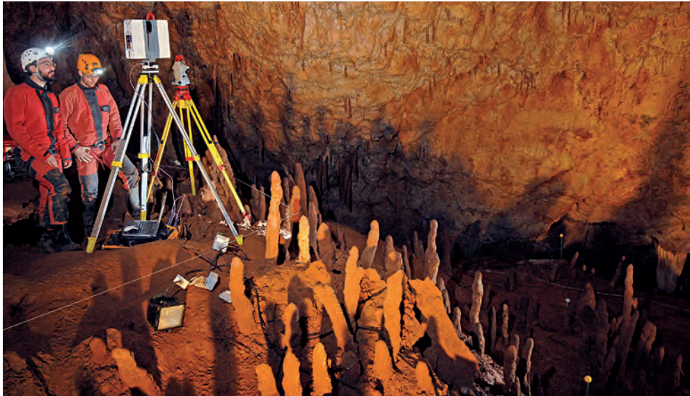
Photo 1 - Acquisition du nuage de points sur le terrain par lasergrammétrie (ici un scanner Leica HDS 6000) et référencement local avec une station totale. Les sphères colorées (en bas à droite) servent à la consolidation des nuages entre eux.
