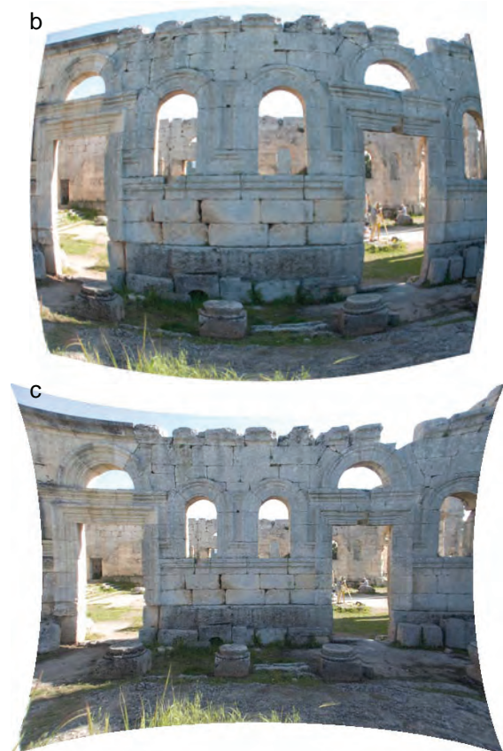
Figure 3 - a) principe de la distorsion optique ; b) distorsion en barillet ; c) distorsion en coussinet.
