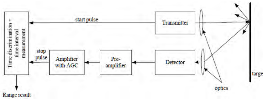
Figure 5 - Schéma des composantes d'un distancemètre à temps de vol (Reshetuyuk, 2009).
