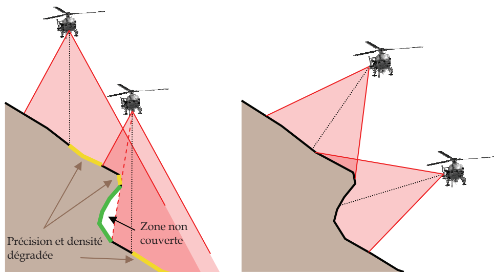
Figure 10 - Acquisition nadirale (gauche) vs oblique (droite) de pentes ou de falaises. La rotation du LiDAR perpendiculaire à la pente permet d'obtenir une précision et une densité homogène. Cela permet également de couvrir les zones surplombantes sans zone d'ombre.
