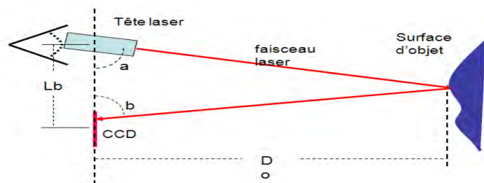
Figure 9 - Principe de mesure de distance par triangulation (@mensi, modifié).
