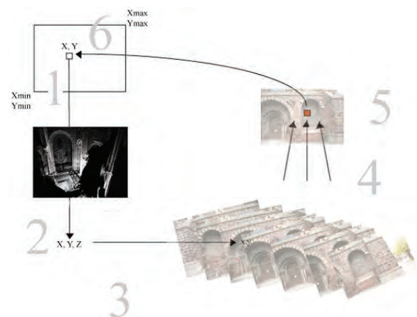
Figure 13 - Processus de calcul d'une orthophoto.
