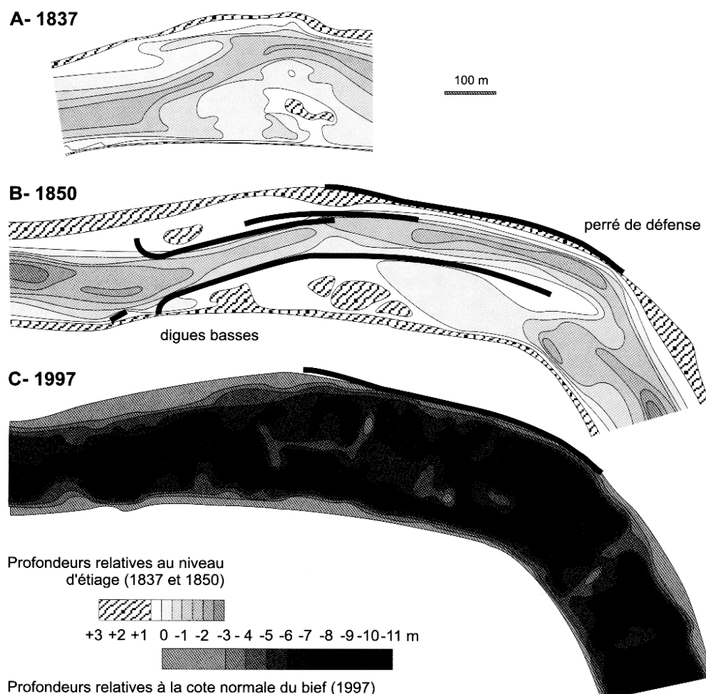
Figure 4 : Bathymétrie du lit mineur de la Saône au niveau du passage des Trois Pierres (Pk 27-28) en 1837 (d'après Plan et profils en travers de la Saône au 1/2 500 e des Passages de l'isle Bène, de la Pradelle et des trois Pierres par le géomètre Chevcoot , en 1850 (d'après Plans et profils en travers de la Saône de Saint-Bernard à Caluire au 1/2 000 e ) et en 1997 (Service Navigation de la Saône, subdivision de Mâcon)
