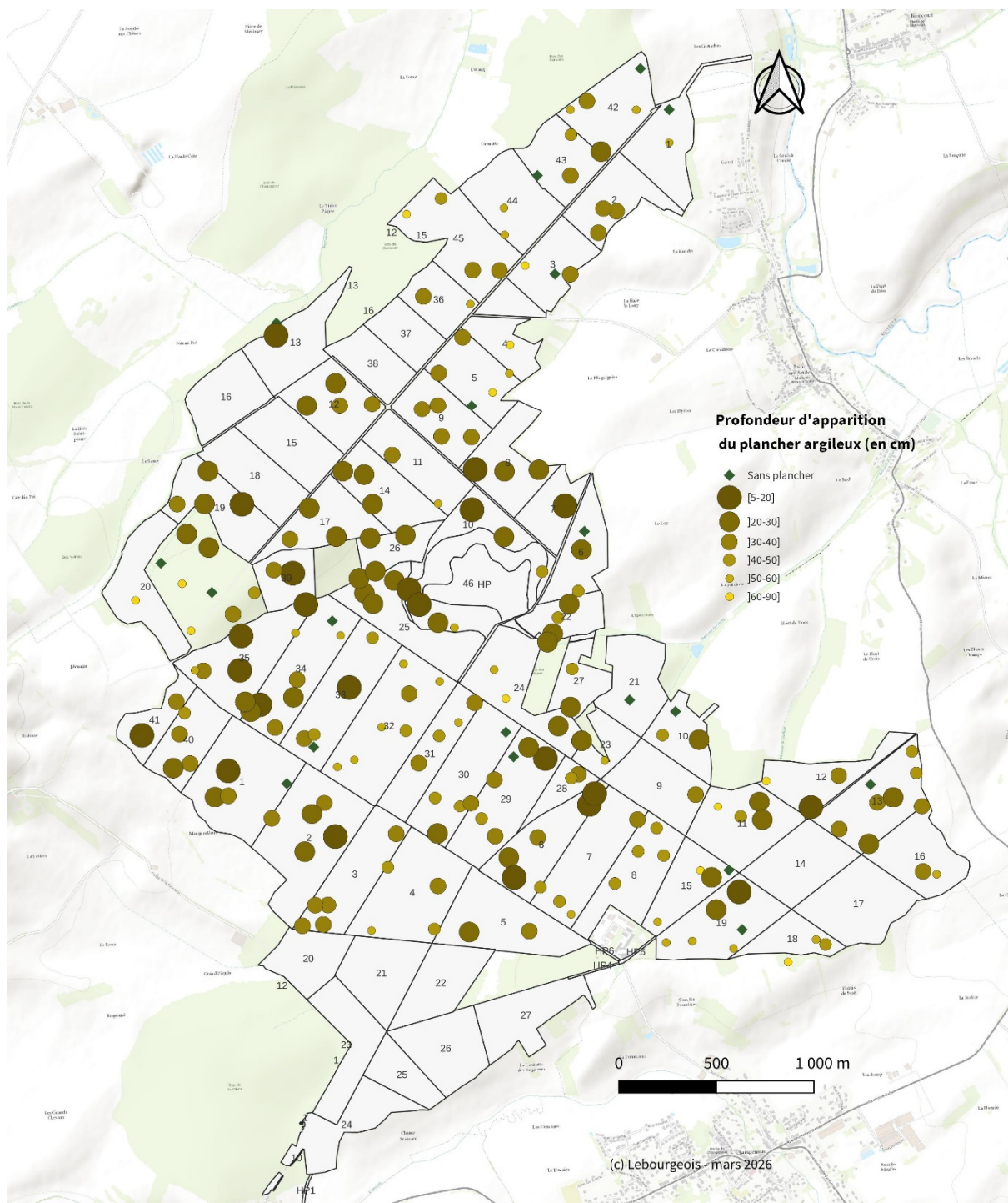
Figure 23 | Cartographie de la profondeur d'apparition d'un plancher argileux (en cm) pour les 213 placettes installées en forêts de Brin et d'Amance.
