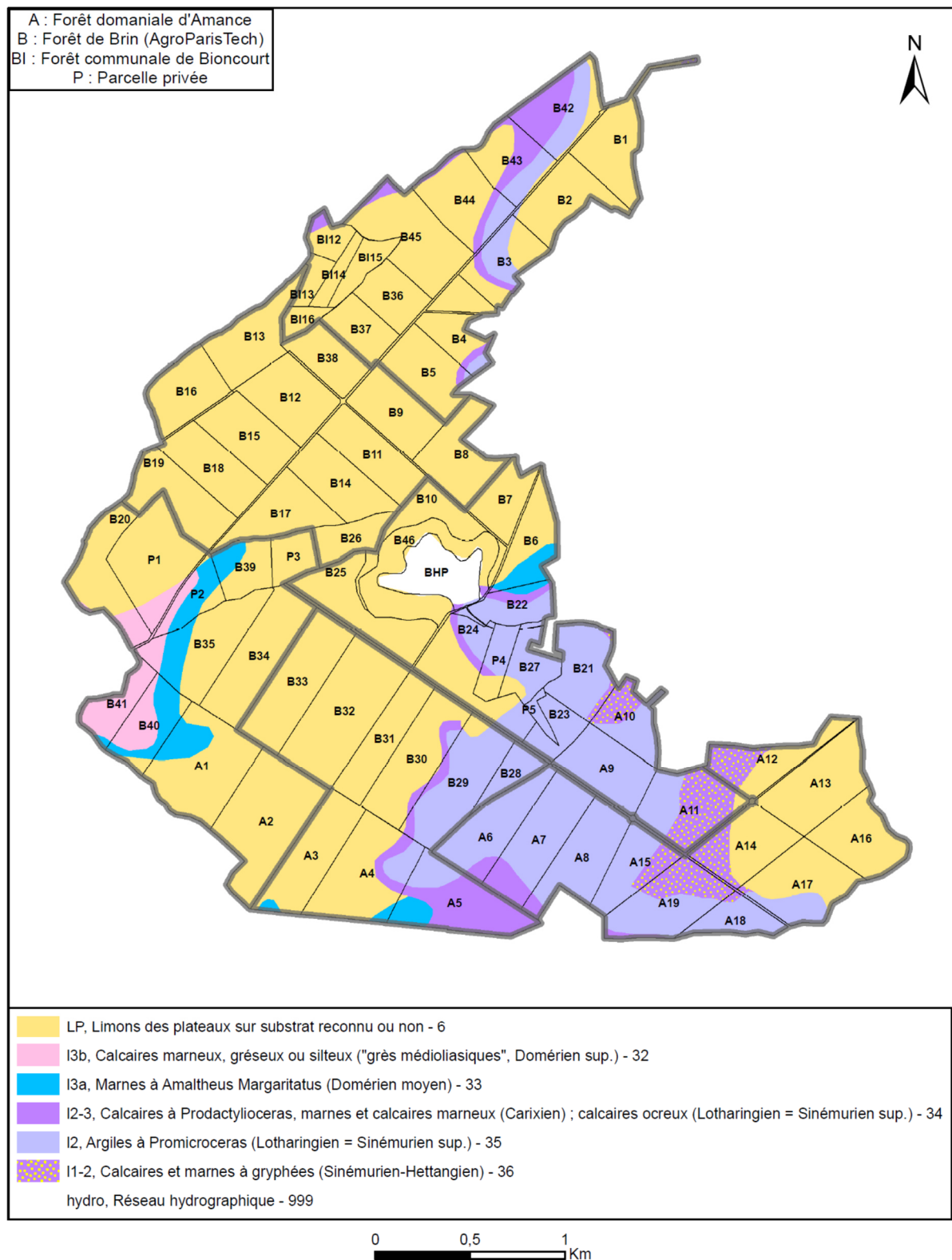
Figure 5 | Carte géologique simplifiée des forêts étudiées (Source AgroParisTech-2021 – C. Bresson). B = Brin ; A = Amance ; P = Privée ; numéro des parcelles.
