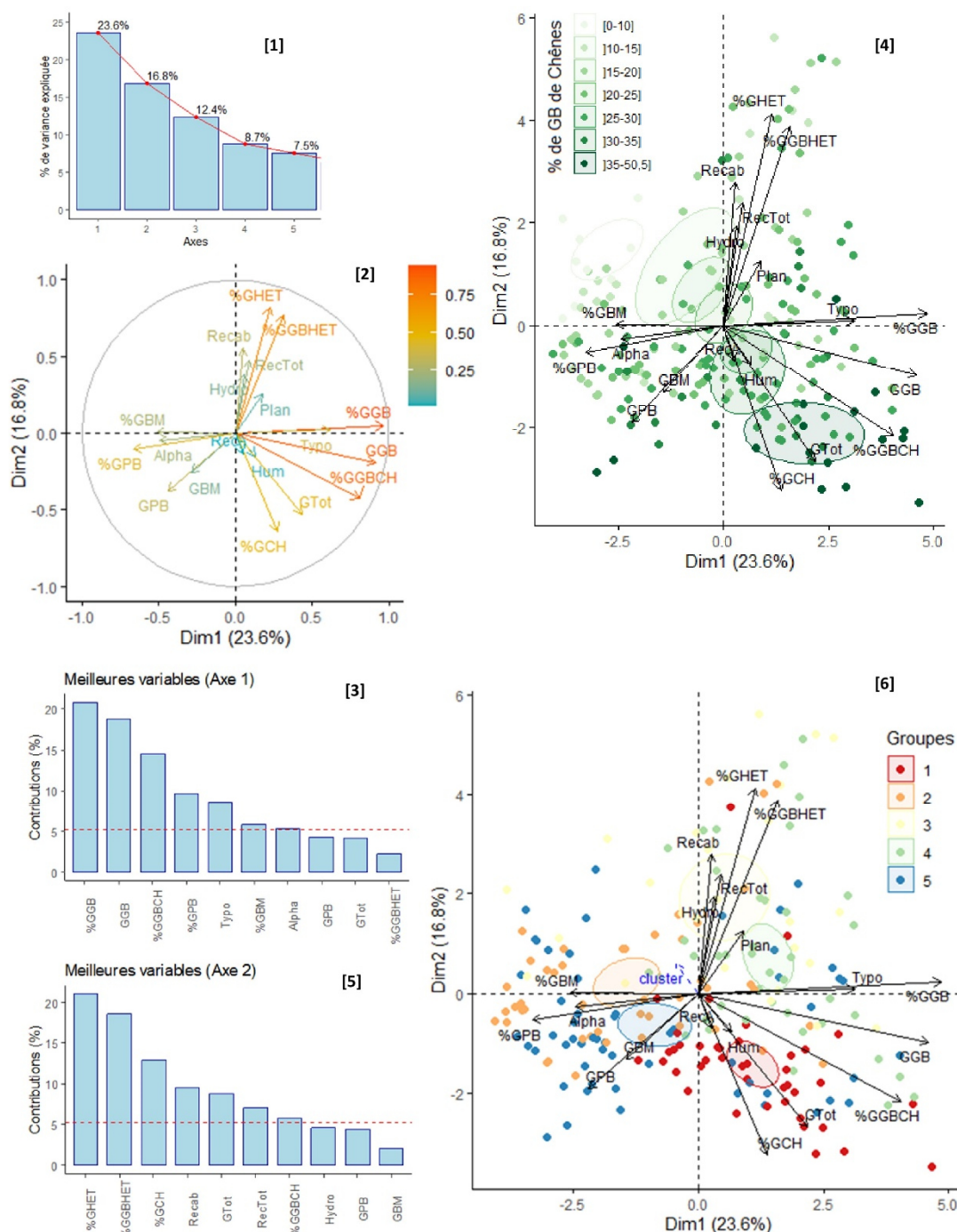
Figure 41 | Résultat de l'analyse en composantes principales effectuée sur les 213 relevés. [1] : % de variance expliquée par les différents axes. [2] : répartition des 20 variables écologique (5) et sylvicole (15) sur le plan factoriel 1-2. La couleur indique l'importance de la variable pour l'explication des axes ( \cos^2 ). [3] : Contributions des 10 meilleures variables à l'interprétation de l'axe 1 (23,6 % de variance expliquée). [5] : Contributions des 10 meilleures variables à l'interprétation de l'axe 2 (16,8 % de variance expliquée). Pour [3] et [5], la ligne rouge en pointillé indique le seuil significatif de la contribution des variables (ici 1/20 \times 100 = 5\% ). [4] : répartition des 213 relevés sur le plan factoriel 1-2. La couleur indique le % de Gros bois de Chênes dans la surface terrière totale (% GGBCH). [6] : Représentation des 5 groupes de relevés issus de la CAH effectuée à partir de l'ACP.
