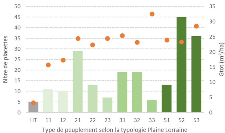
Figure 36 | Nombre de placettes selon les types de peuplements dans les forêts de Brin et d'Amance selon la typologie de la Plaine lorraine. 1 = petit bois ; 2 = bois moyen ; 3 = gros bois et 5 = irrégulier. Les ronds orange correspondent à la surface terrière totale moyenne (Gtot en m²/ha) par type. HT = Hors typologie, Gtot < 7 m²/ha ou pas d'arbres précomptables.
