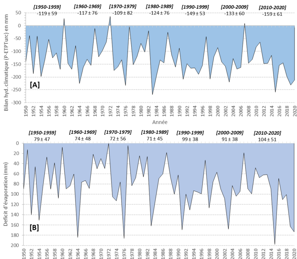
Figure 4 | Évolution du bilan hydrique climatique (P-ETPTurc) [A] et du déficit d'évaporation (ETR-ETP) [B] sur la période 1950 à 2020. L'évapotranspiration potentielle a été calculée avec la formule de Turc. Le déficit d'évaporation a été calculé à partir du modèle de bilan hydrique de Thornthwaite et Mather (1955). Pour le calcul, une réserve utile du sol de 120 mm (sur 70-80 cm) a été considérée selon les résultats des descriptions pédologiques (voir partie résultats : texture LA sur Argile ; plancher à 40 cm ; traces d'hydromorphie à partir de 27 cm ; enracinement fort avant le plancher et moindre après). Cette RU est sans doute sous-évaluée pour les Chênes mais semble raisonnable pour les Hêtres beaucoup plus sensibles aux contraintes d'engorgement que les chênes (enracinement nettement moins profond dans ces contextes). Les données en gras correspondent aux moyennes et écarts-types pour chaque période de 10 ans.
