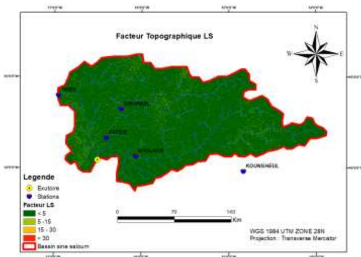
Figure 4 : Facteur topographique LS du Sine Saloum
