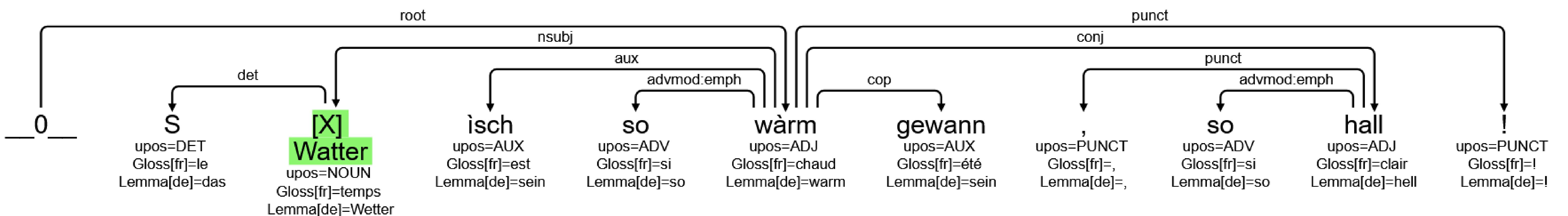
Corpus UD_Alemannic-DIVITAL
