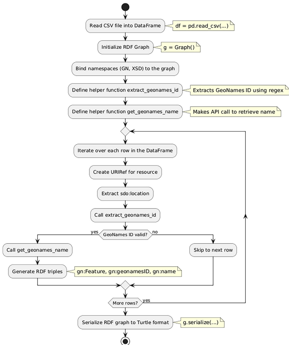
Fig. 3. Geonames Converter Pipeline.
