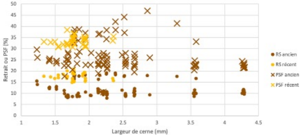
Fig. 1 : Évolution du RS et du PSF en fonction de la largeur de cernes des deux Chênes
