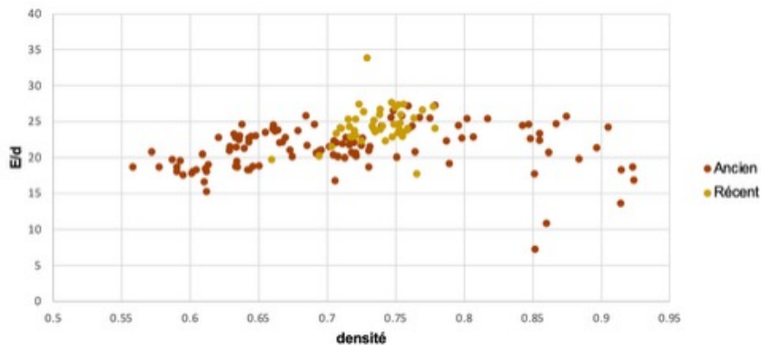
Fig. 3 : Évolution du E/d en fonction de la densité des deux lots de Chênes
