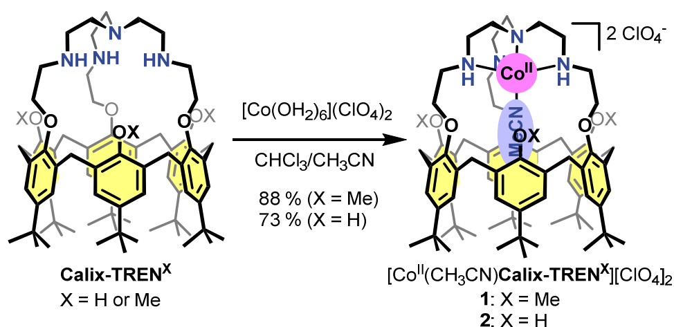
Scheme 1. Synthesis of funnel complexes [\text{Co}^{\text{II}}(\text{CH}_3\text{CN})\text{Calix-TREN}^{\text{Me}}][\text{ClO}_4]_2 ( 1 ) and [\text{Co}^{\text{II}}(\text{CH}_3\text{CN})\text{Calix-TREN}^{\text{H}}][\text{ClO}_4]_2 ( 2 ).
