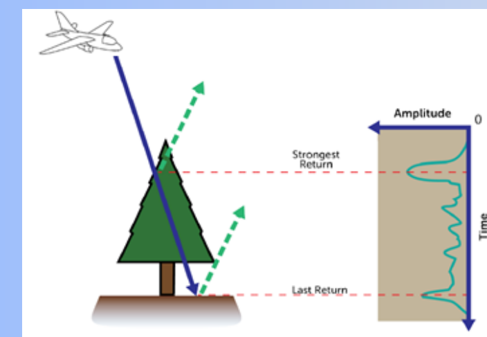
Figure 17. Croquis conceptuel de la trajectoire du rayonnement d'un LiDAR et son comportement en terme de fréquence.
