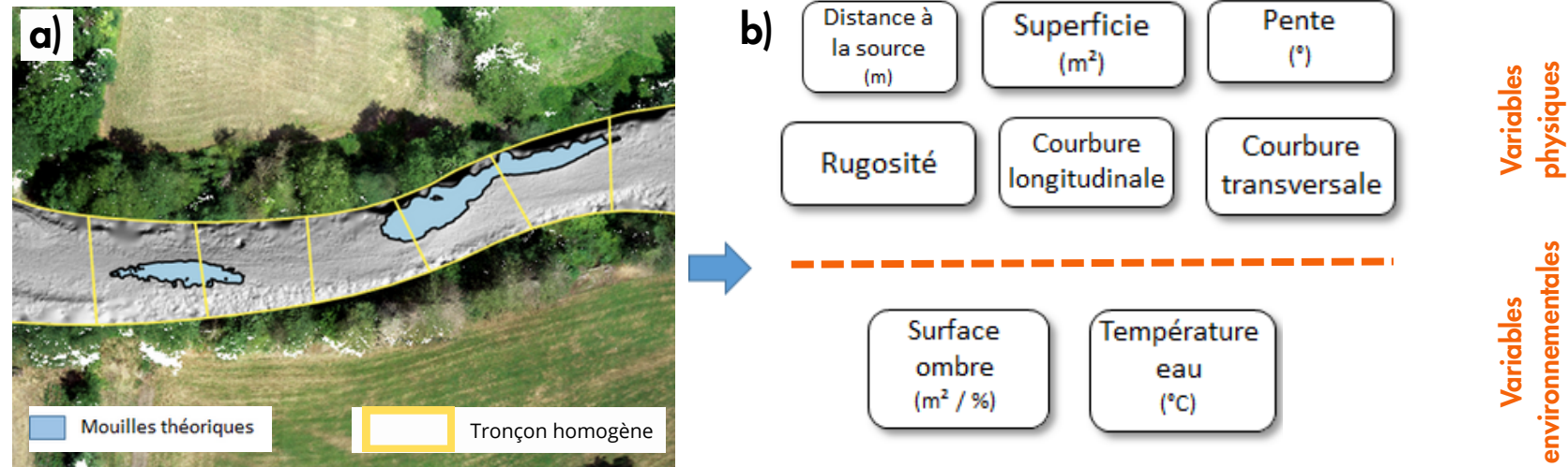
Figure 31. a) échelle d'extraction des variables par tronçon de 20m, b) typologie des variables extraites
