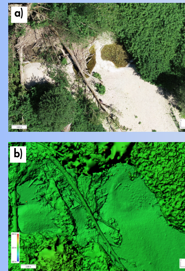
Figure 16. Extrait de divers faciès composés de débris ligneux, embâcles, végétation alluviale, banc de galets, a) Orthophoto, b) Modèle numérique de surface
