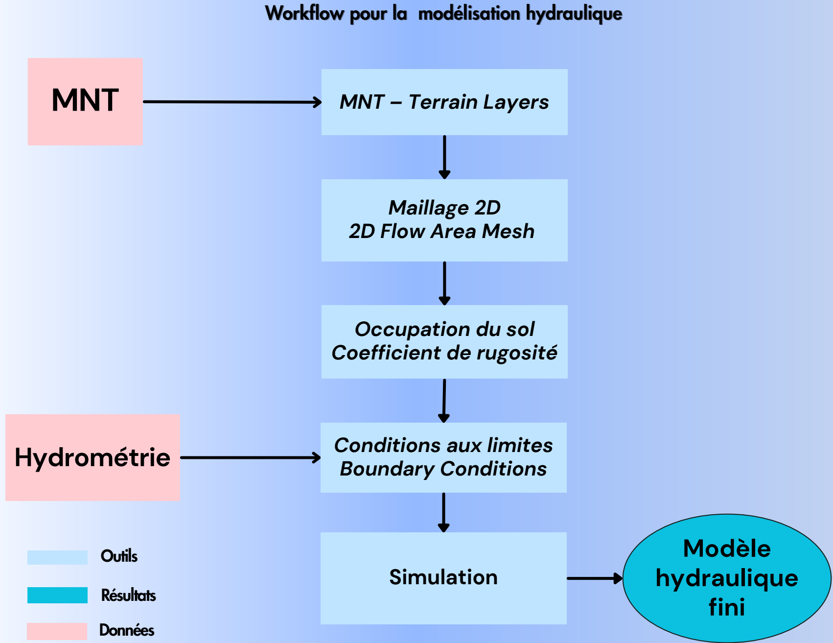
Figure 30 : Organigramme de la chaîne de traitement par méthode hydraulique
