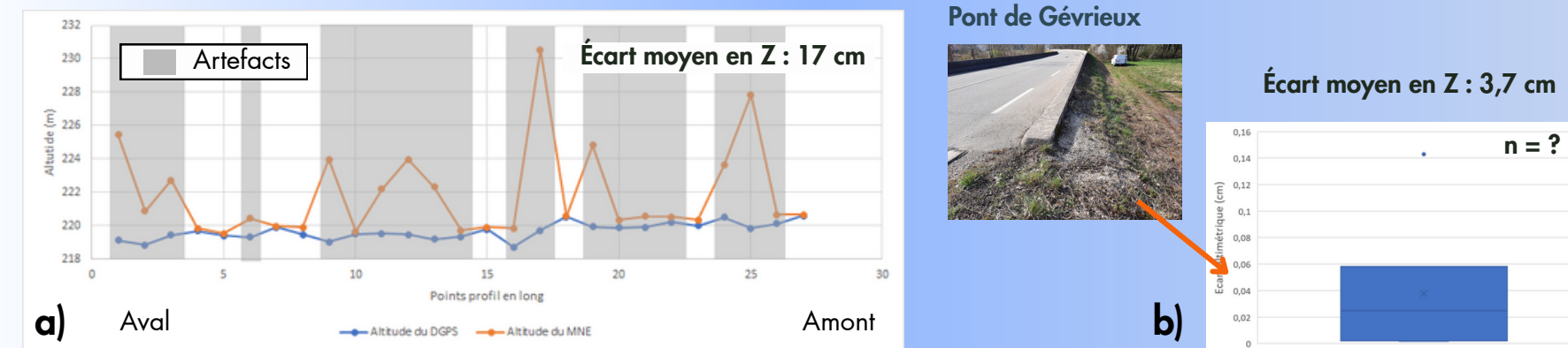
Figure 22. a) Comparaison entre profil en long altimétrie SfM et altimétrie DGNSS, b) Écart entre altimétrie SfM et point de contrôle in-situ DGNSS, site 1 - mission du 25/03/2022
