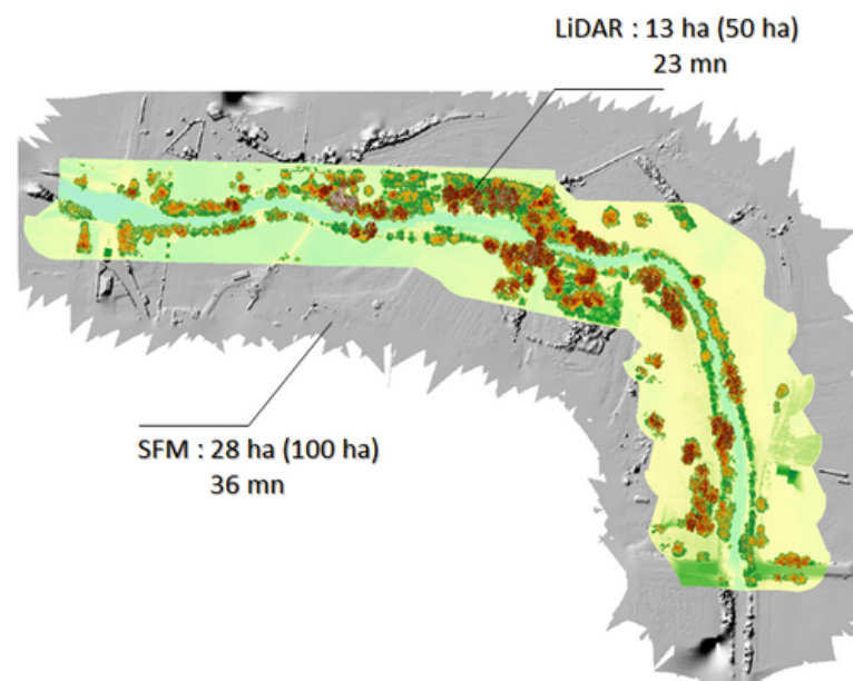
Figure 45. Surfaces couvertes par la SfM et le LiDAR pour un même linéaire, exemple du site 2.
