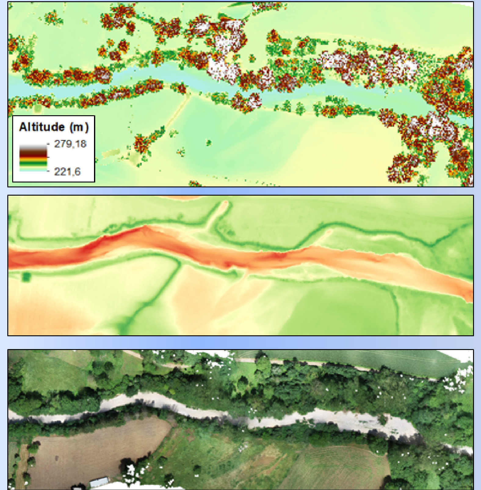
Figure 20. a) Modèle Numérique de surface (MNS), b) Modèle Numérique de Terrain (MNT), c) Orthomosaïque - extrait du site 2 (Lejot J. et al. , 2023)
