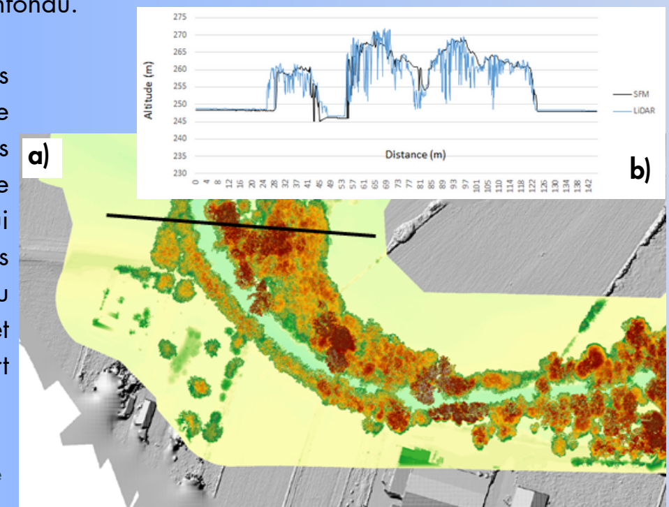
Figure 47. a) Extrait d'un MNS par méthode SfM & LiDAR, b) transect de comparaison entre les deux méthodes.
