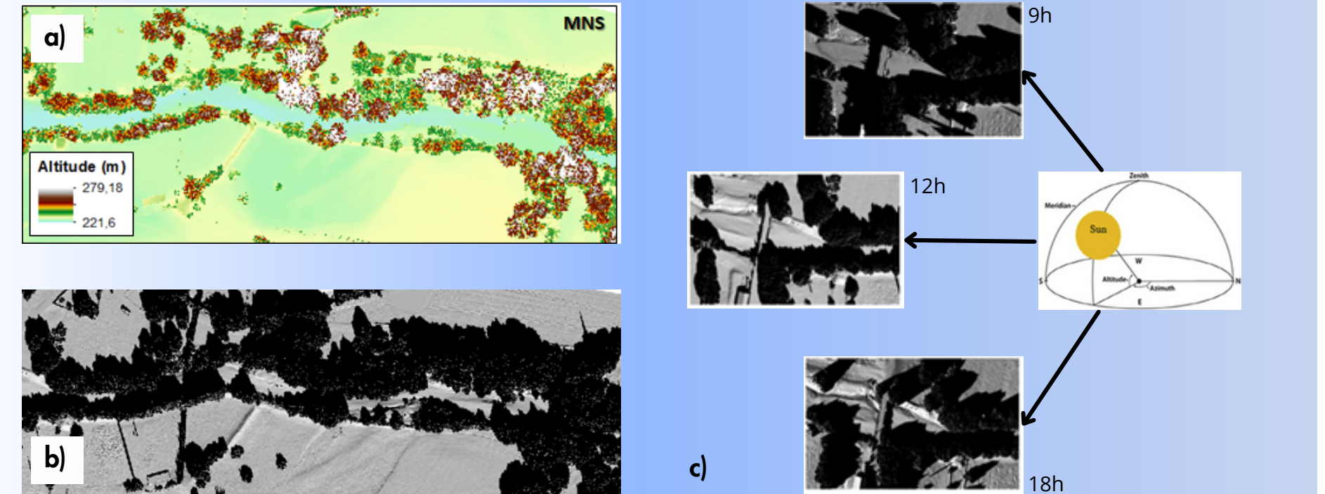
Figure 32. a) extrait d'un MNS - site 2 et b) sa carte d'ombrage, c) Simulation d'ensoleillement à différents pas horaire selon un angle zénithal et azimutal
