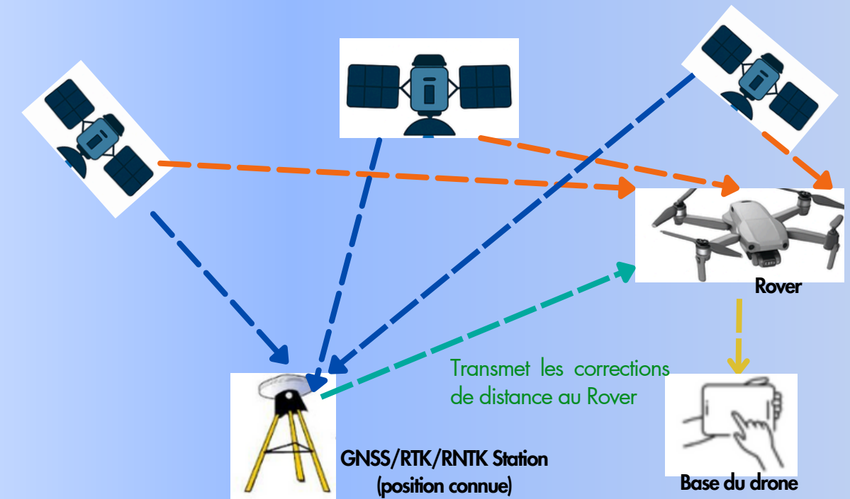
Figure 4 : Architecture d'un positionnement GNSS différentiel pour la géolocalisation centimétrique des données aériennes, relation fonctionnelle entre le récepteur mobile RTK (rover) embarqué sur le drone et la station de référence fixe au sol.
