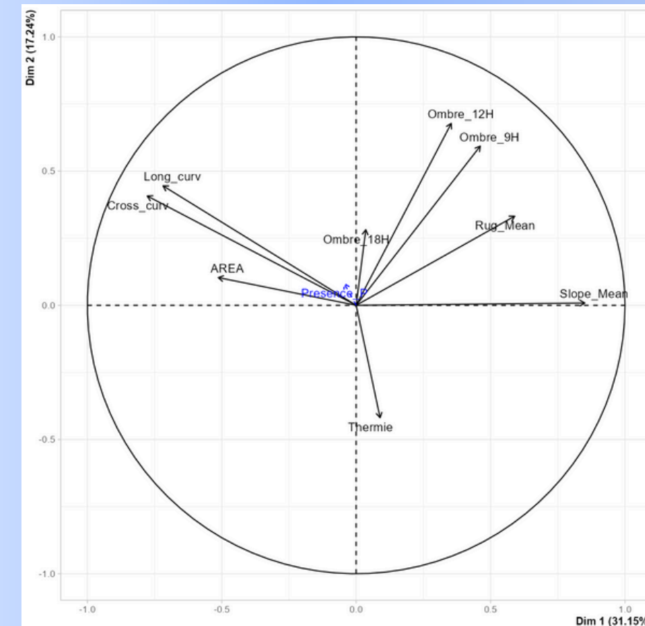
Figure 38. Test du poids des variables physiques et environnementales sur la présence de poisson dans les zones de refuges.
