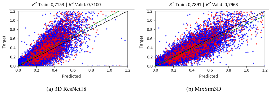
FIGURE 3 : Graphiques de dispersion des résultats après ajustement des modèles 3D ResNet18 (a) et MixSim3D (b). Les points bleus correspondent aux échantillons du jeu d’entraînement, et les points rouges représentent les échantillons du jeu de validation. La ligne verte est la ligne de régression estimée et la ligne noire est l’identité idéale ( y = x ).
