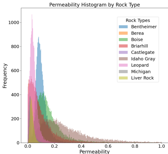
FIGURE 2 : Histogramme de perméabilité pour les 9 types de roche considérés.
