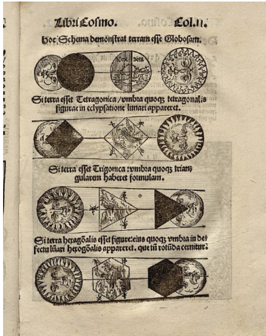
Légende : Différentes ombres portées de la Terre sur la Lune lors des éclipses de Lune, selon la forme envisagée de la Terre. Extrait de Cosmographicus Liber (1524) de Petrus Apianus. (Libre de droits)
