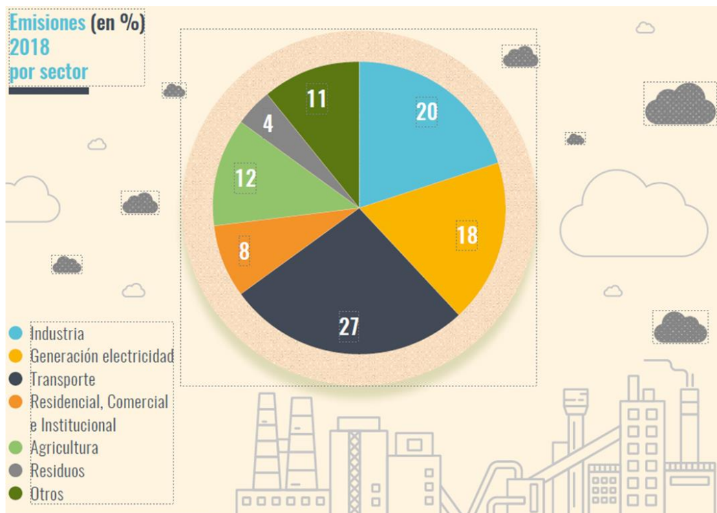
Fig 1. Emisión de GEI por sector en 2018
