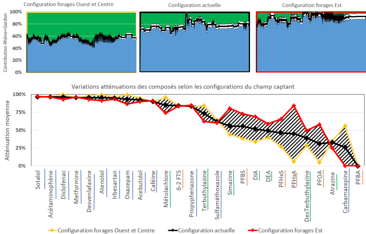
Figure 2 : Atténuations moyennes en sortie d'usine pour les composés pharmaceutiques (bleu), phytosanitaires (vert), industriels (orange) pour la configuration actuelle du champ captant (noir) et des configurations alternatives (rouge, les forages Est sont les plus exploités et jaune, les forages Ouest).
