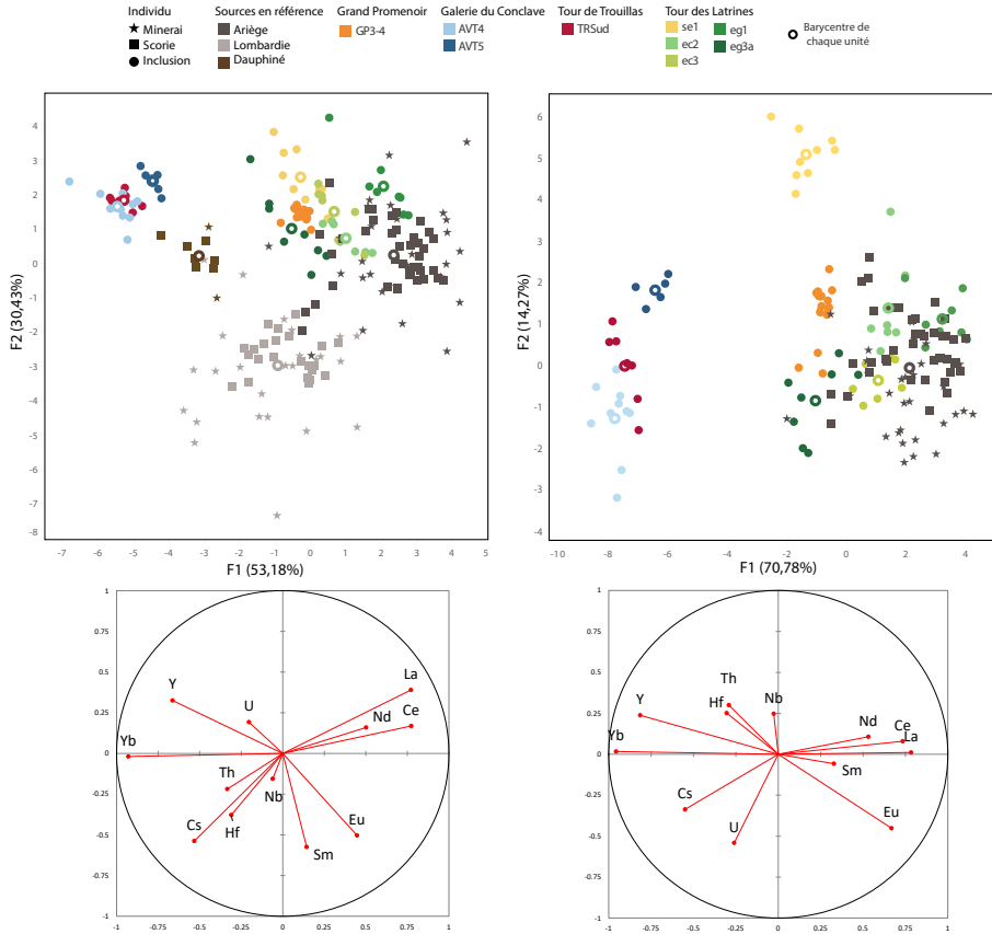
FIG. 3 : Projections sur le premier plan discriminant des résultats de l'analyse discriminante. Deux analyses sont réalisées ; la première (gauche) incluant toutes les classes, la deuxième (droite) focalise l'analyse sur la comparaison Ariège-fers.
