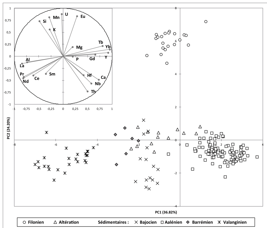
FIG. 2 : Projection, sur le plan défini par les deux premiers facteurs d'une ACP, des individus (scories et minerais) du corpus lorrain. La symbologie représente le type de minerai associé à l'individu.
