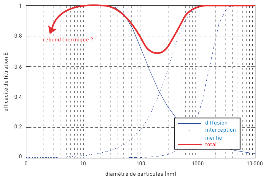
FIGURE 1 Efficacité d'un filtre à fibres Fibrous filter efficiency
