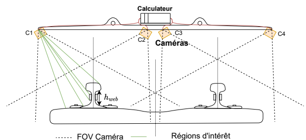
FIGURE 2 – Placement des caméras linéaires.
