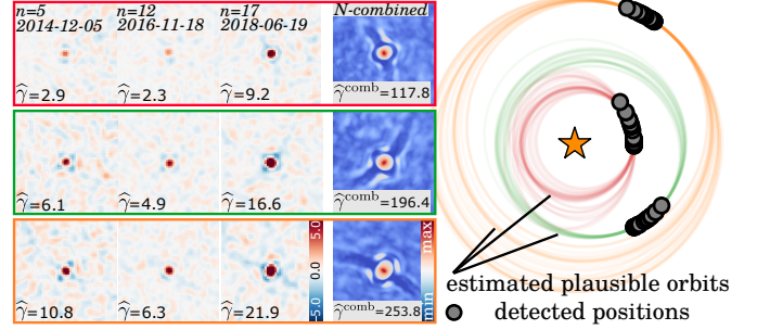
FIGURE 4 : Fusion de 23 observations de l'étoile HR 8799. Gauche : Exemples de cartes de détections individuelles \hat{\gamma} et fusionnées \hat{\gamma}^{\text{comb}} centrées sur les trois exoplanètes connues. Droite : Orbites \hat{\mu} estimées conjointement à la détection.
