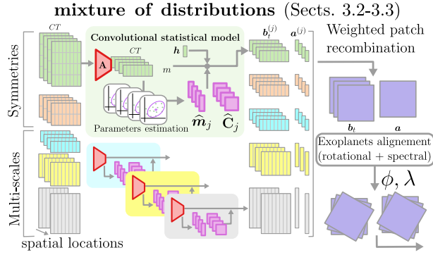
FIGURE 2 : Approche proposée combinant paramètres estimés et apprenables. Elle exploite la diversité spectrale des observations \mathbf{y} via un modèle convolutionnel de mélange de distributions capturant les symétries et les corrélations de la nuisance à différentes échelles spatiales. Le réseau f_\nu (U-Net) apprend un a priori sur l’objet pour filtrer le score de détection \hat{\gamma} issu du modèle statistique.
