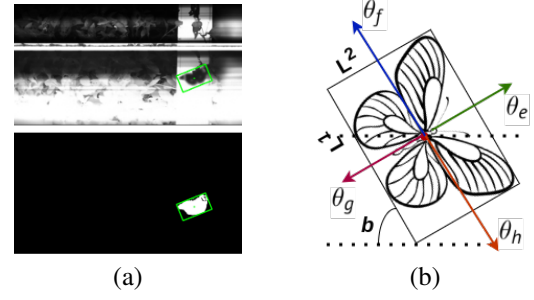
FIGURE 3 : Phase de détection : (a) Masque issu de la détection (b) Mesures de pré-observation sur un OBB.
