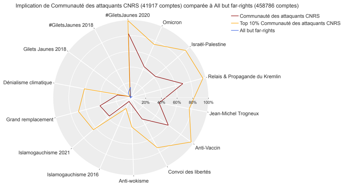
FIGURE 5 – Contribution de la communauté numérique étendue (41,9k comptes) sur la période 2022-2023 des 80 comptes ayant attaqué OpenPortability à différentes polémiques de la twittosphère française depuis 2018.
